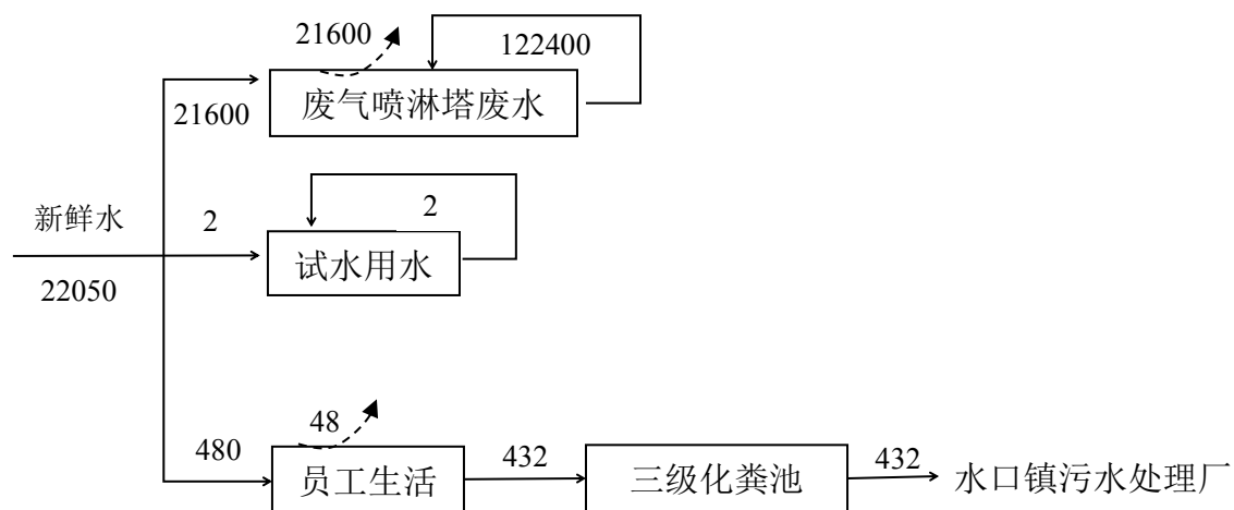
图 1-1 项目水平衡图 (m³/a)
