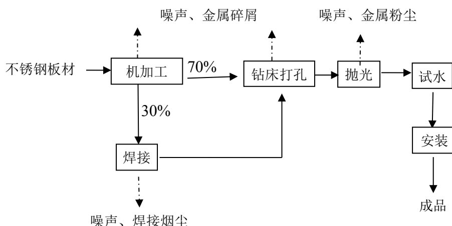
图 5-1 生产工艺流程及产污环节示意图
