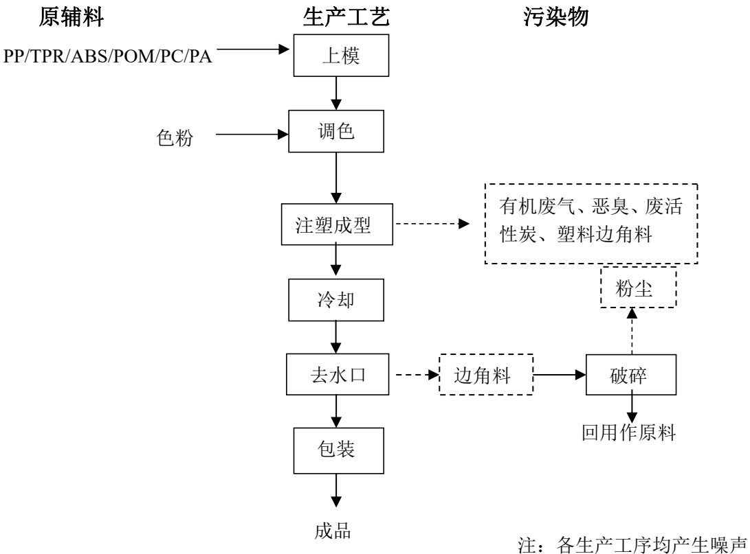
图 5-1 塑料制品生产工艺流程图
