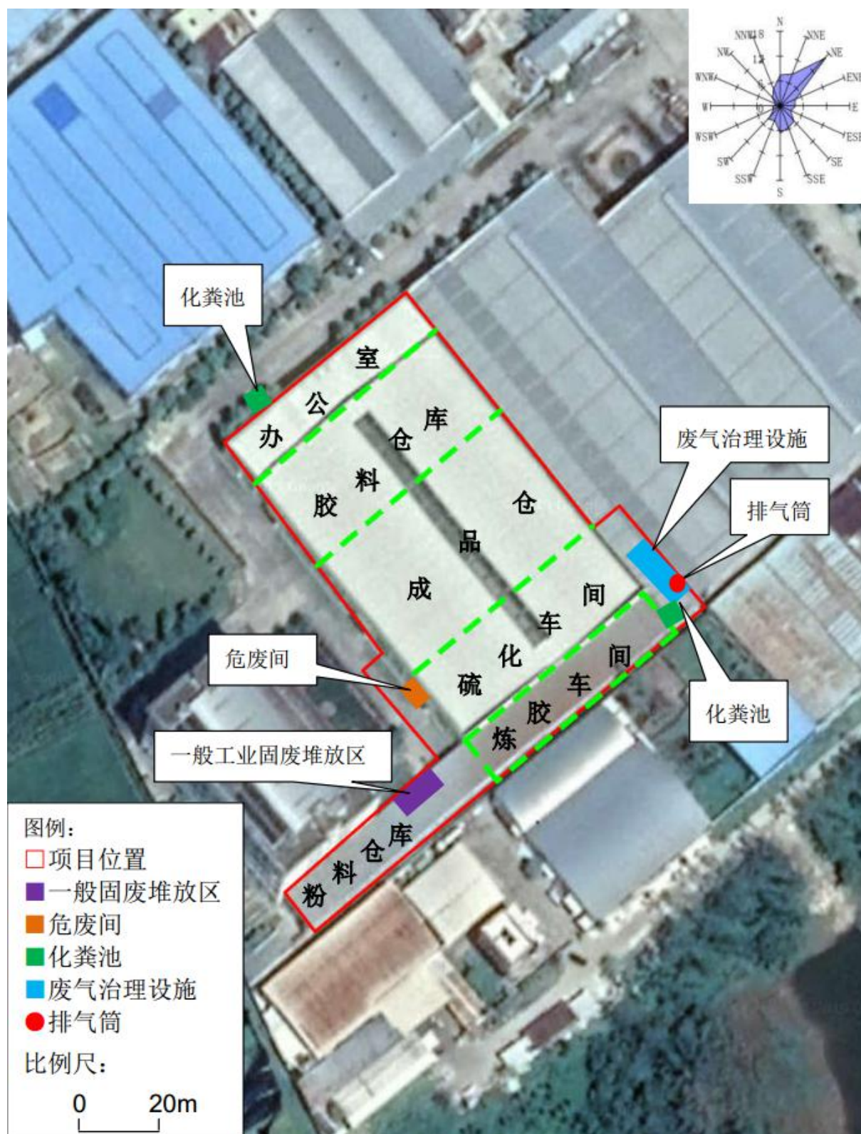
图 2.1-6 整改后项目平面布置图
