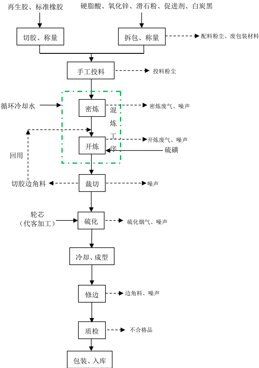
图 3.1-1 橡胶制品产品生产工艺和产污节点图
