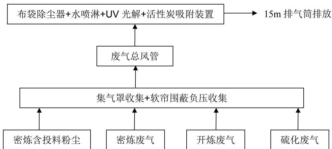
图 7.2-1 本项目拟采取的废气治理工艺
