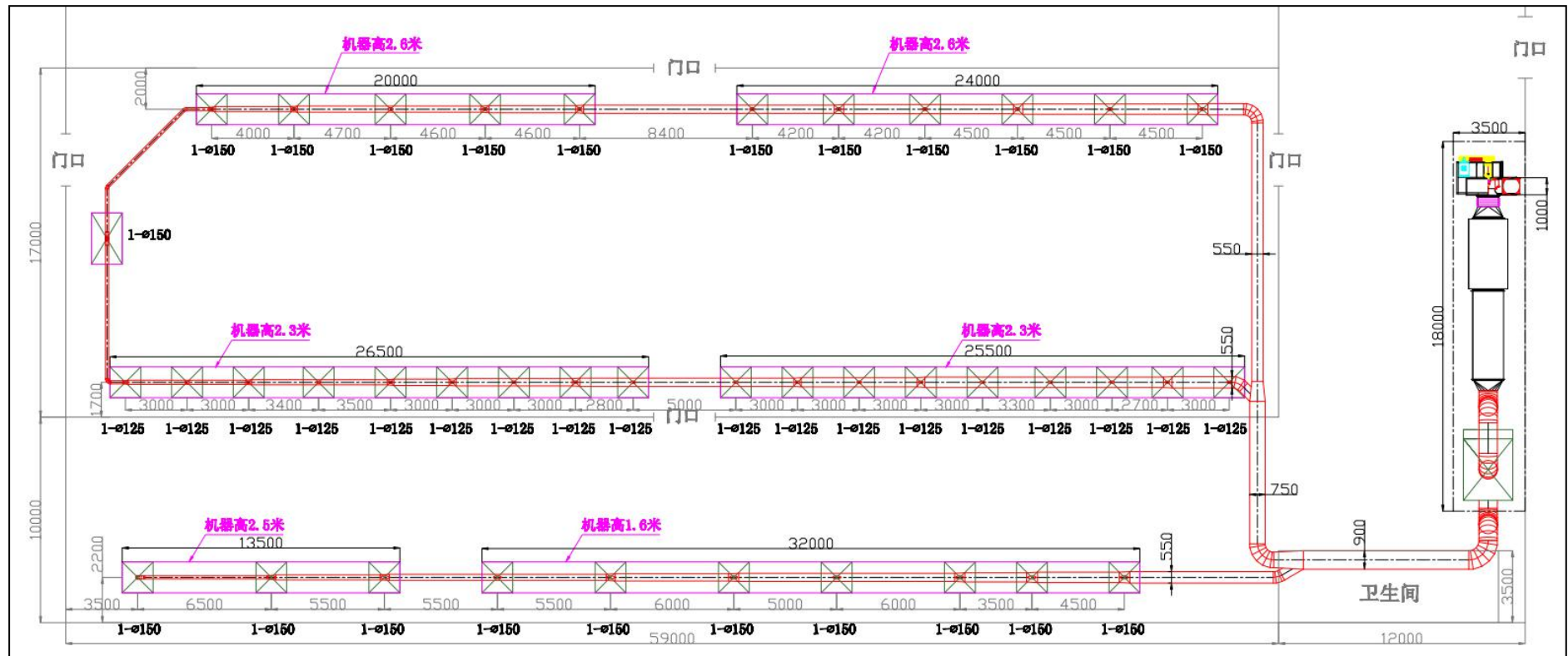
图 7.2-1 废气收集和输送管网设计图
