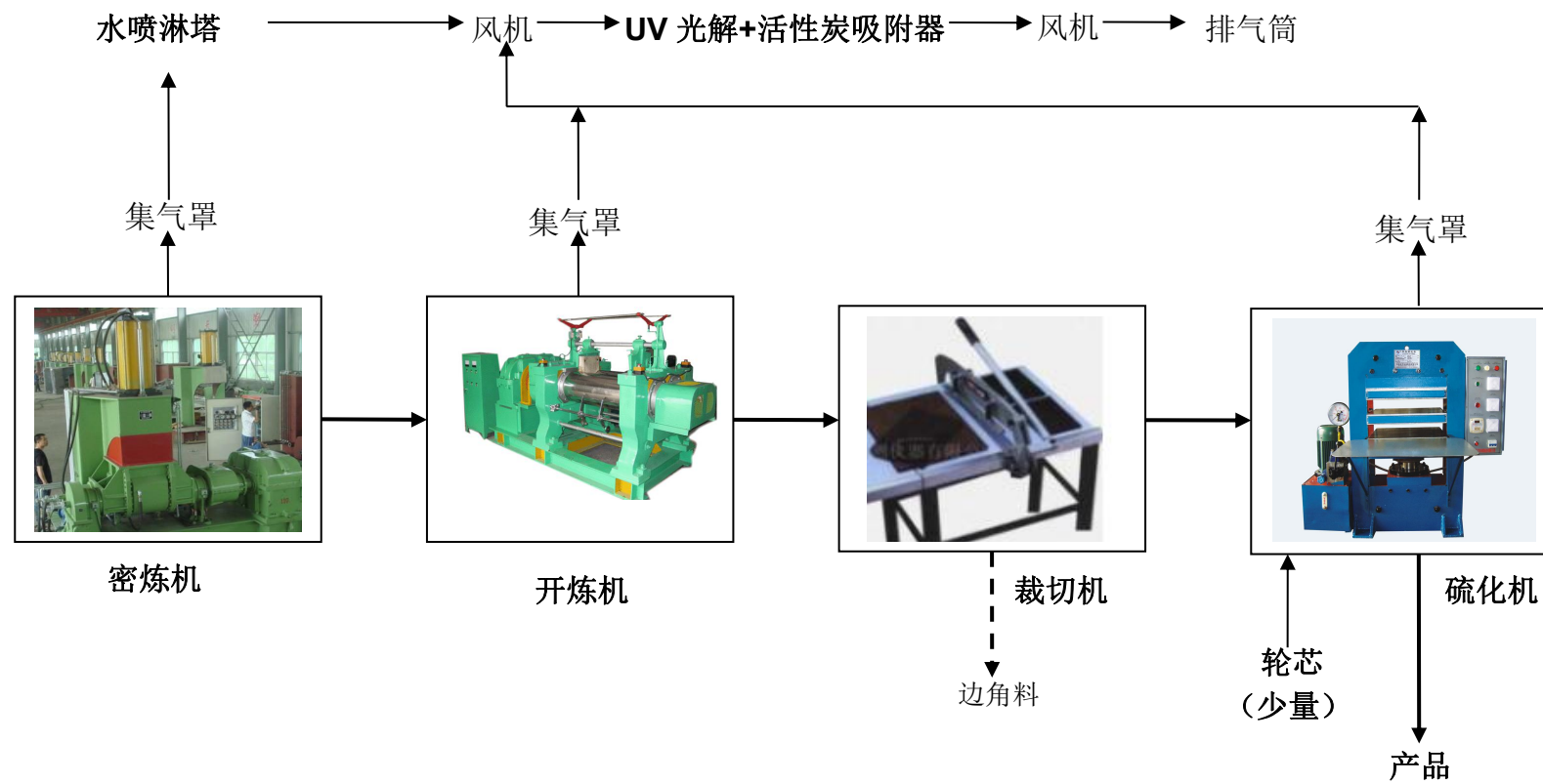
图2.1-9 生产设备工序连接及废气收集示意图（现有工程）
