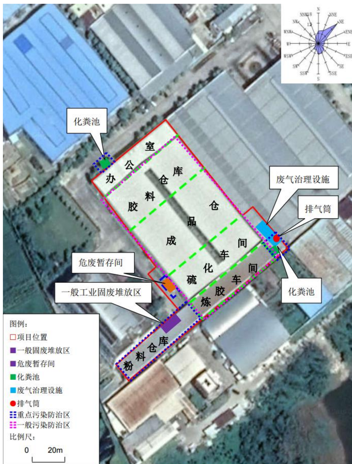
图 7.5-1 项目地下水分区防治图
