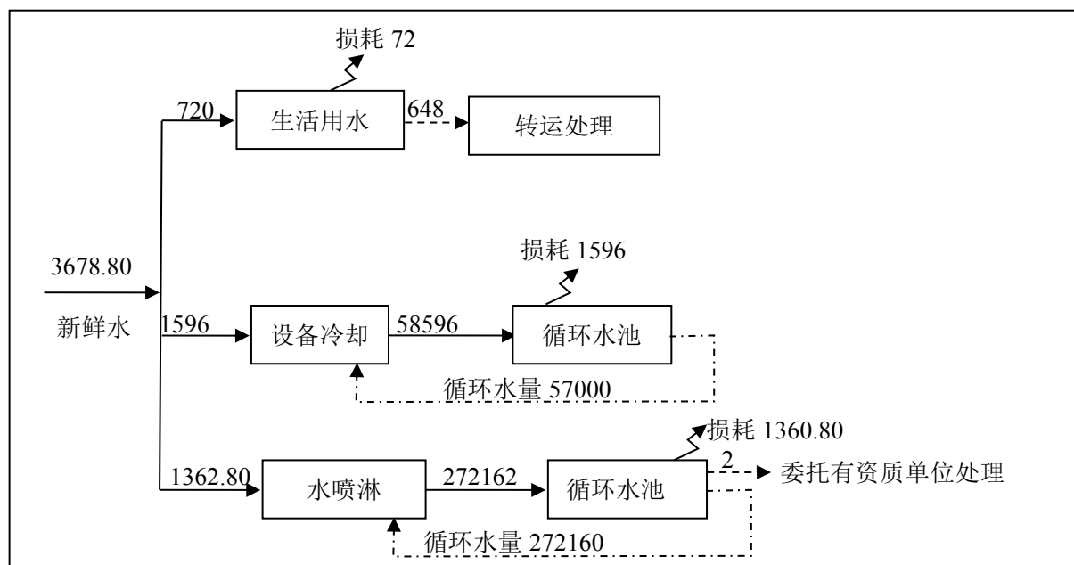
图 3.2-1 已建工程水平衡图 (单位: m 3 /a)
