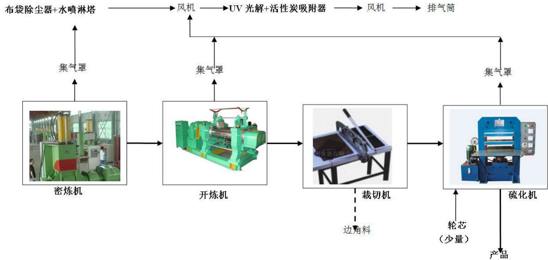
图2.1-10 生产设备工序连接及废气收集示意图（整改工程）
