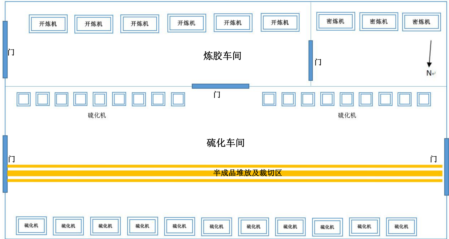
图 2.1-7 项目生产车间设备平面布置图
