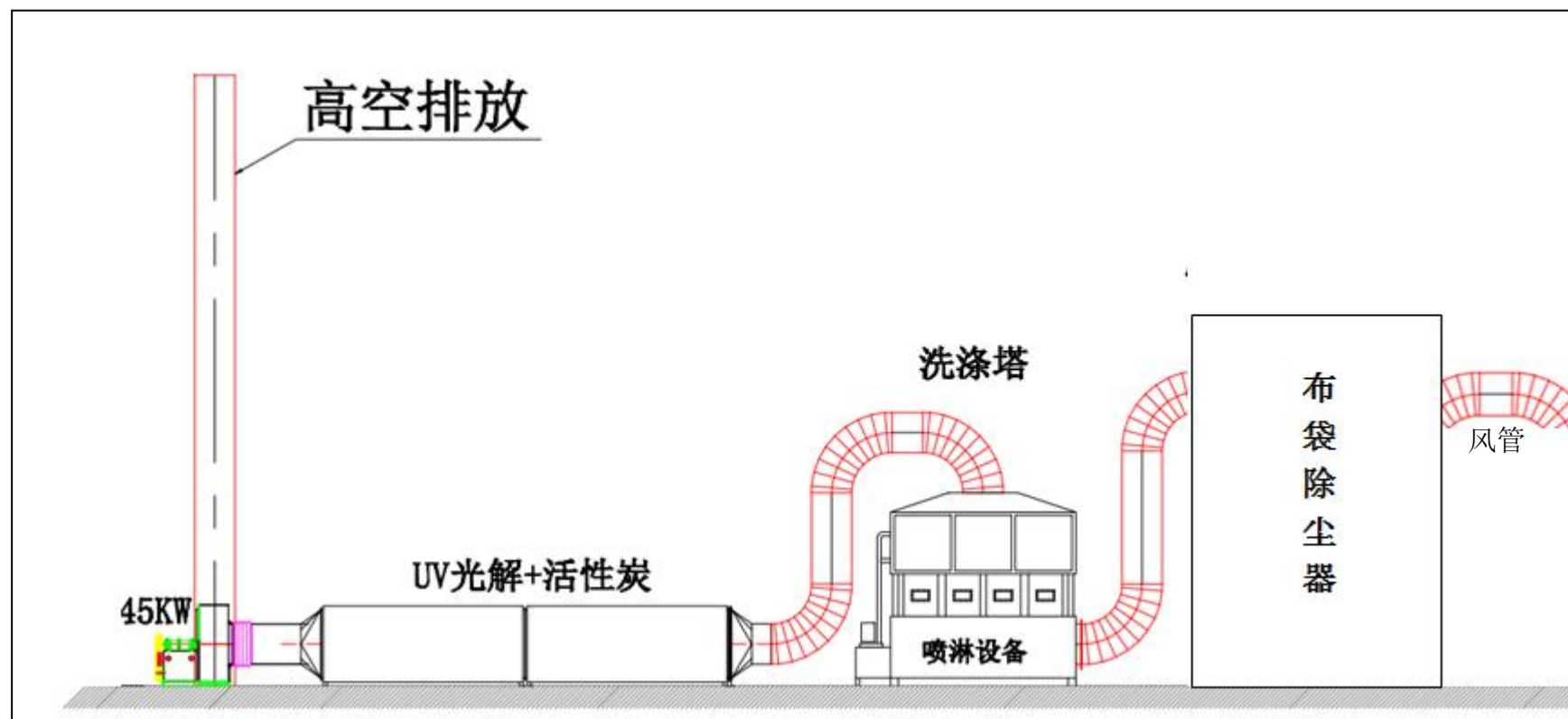
7.2-2 废气治理设施连接图
