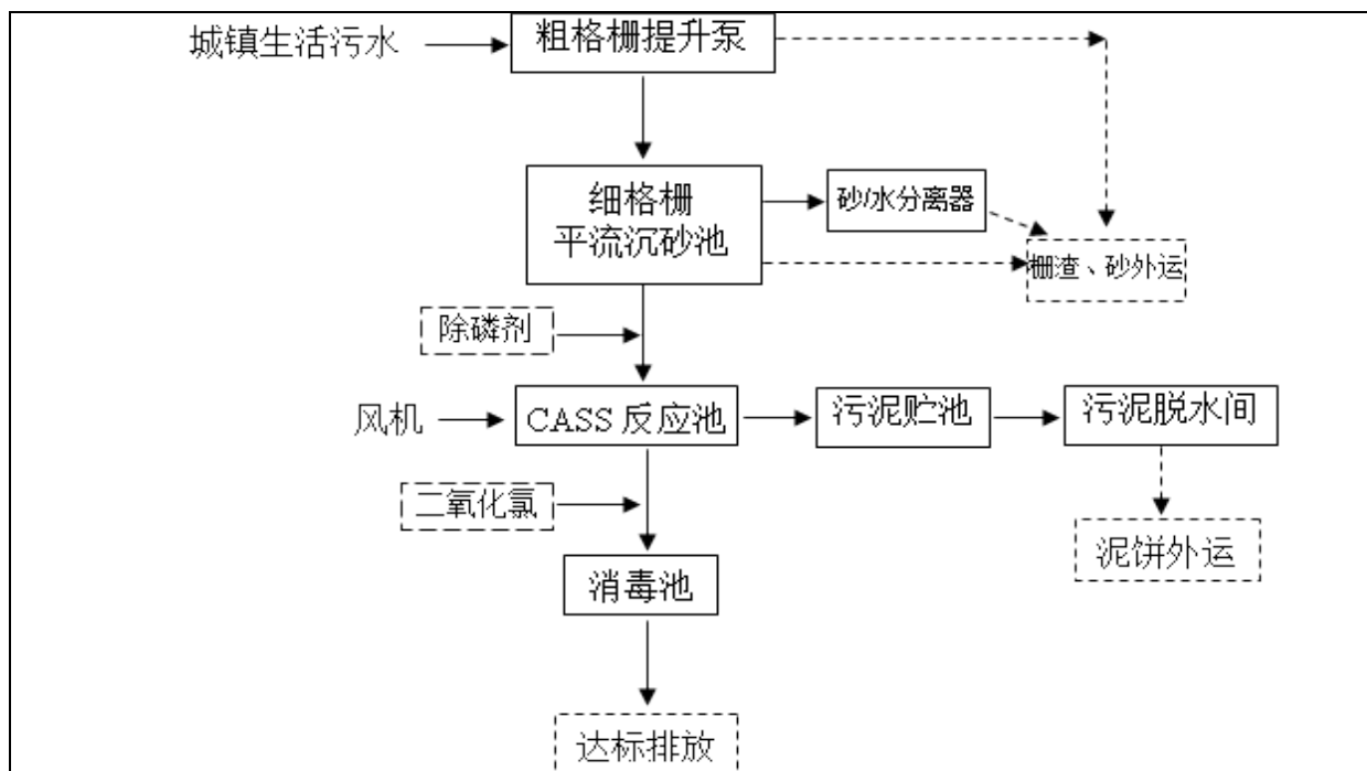
图 7-1 污水处理厂处理工艺流程
