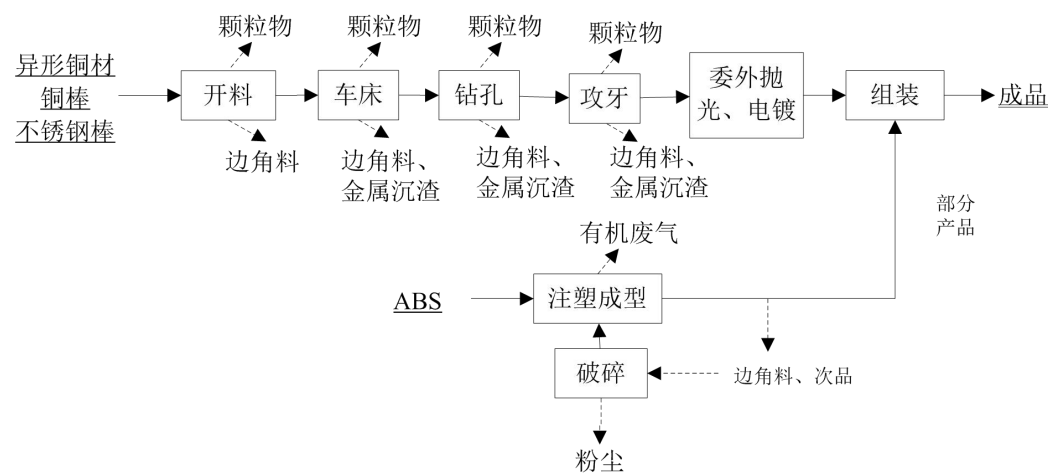
图6-1 铜铰链、铰链装饰盖生产工艺流程图
