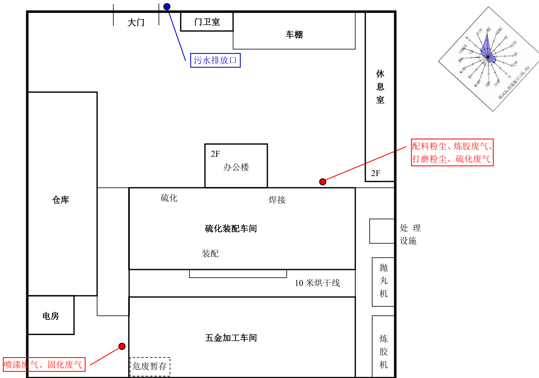
图 3.3-4 项目平面布置图
