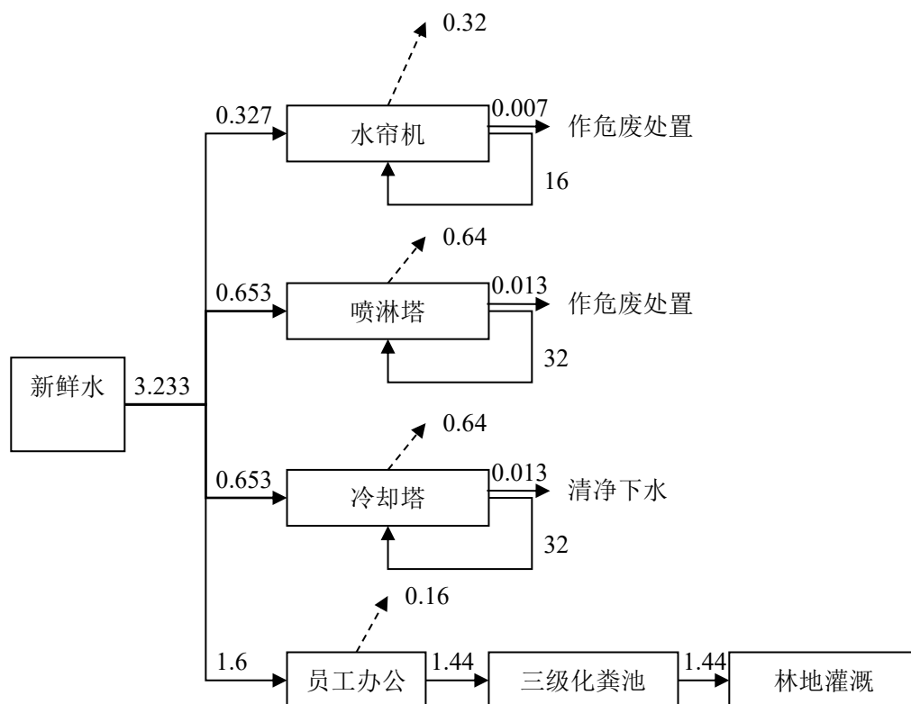
图 3.9-3 项目水平衡图（单位：m 3 /d）
