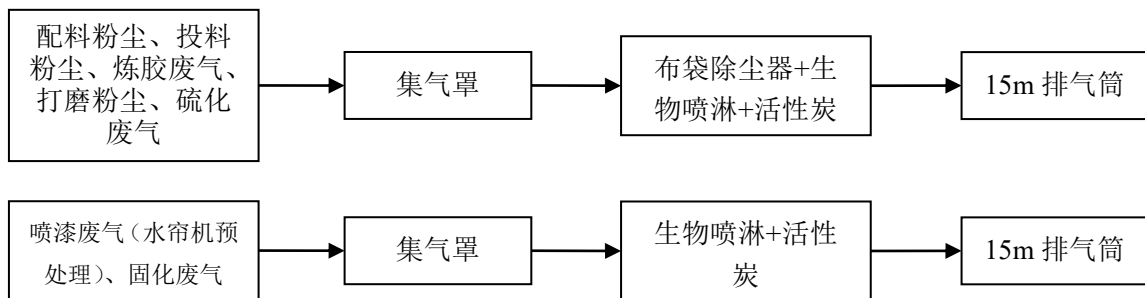
图 6.2-1 项目有机废气收集、处理流程
