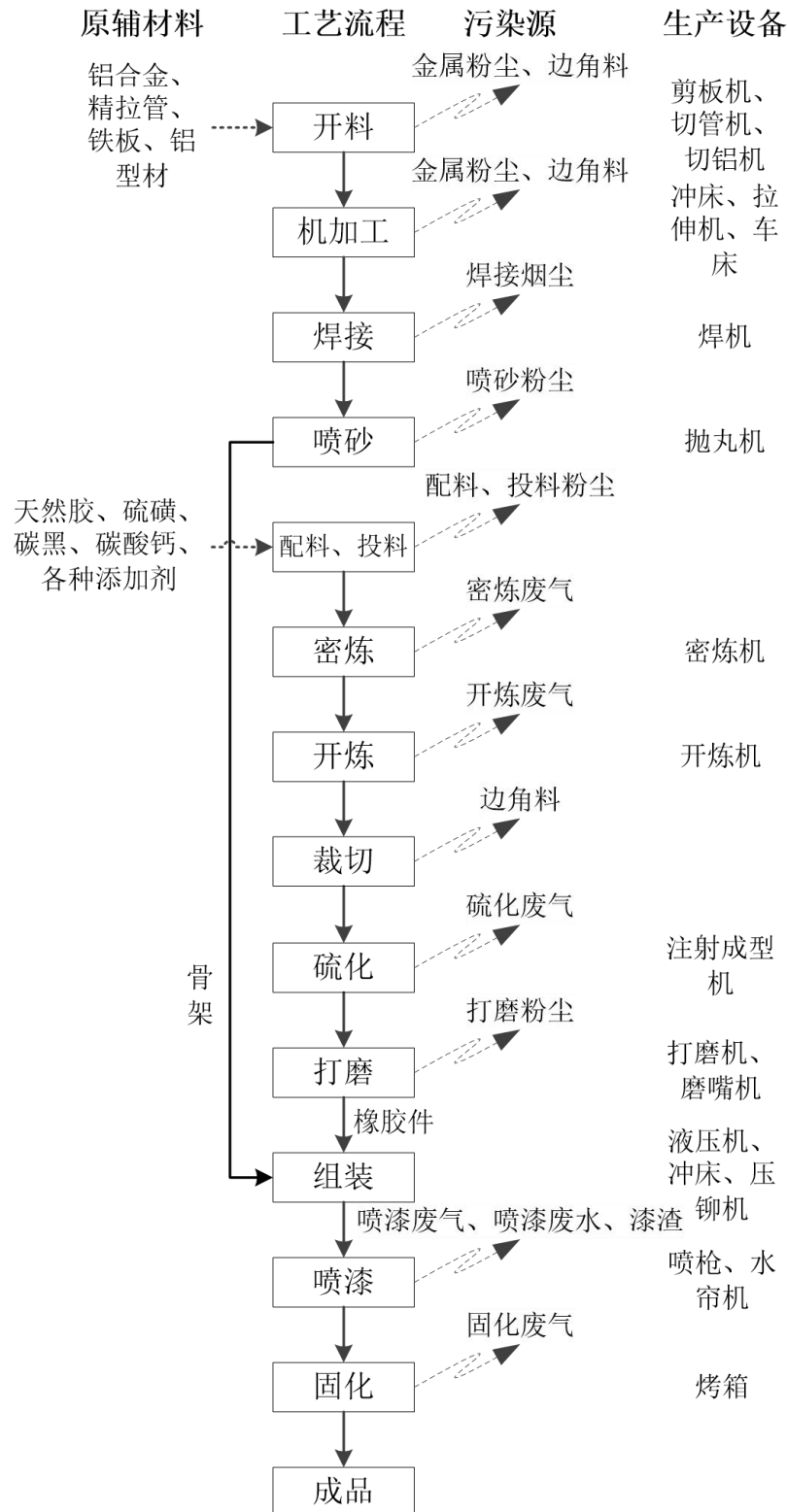
图 3.8-1 项目生产工艺流程图
