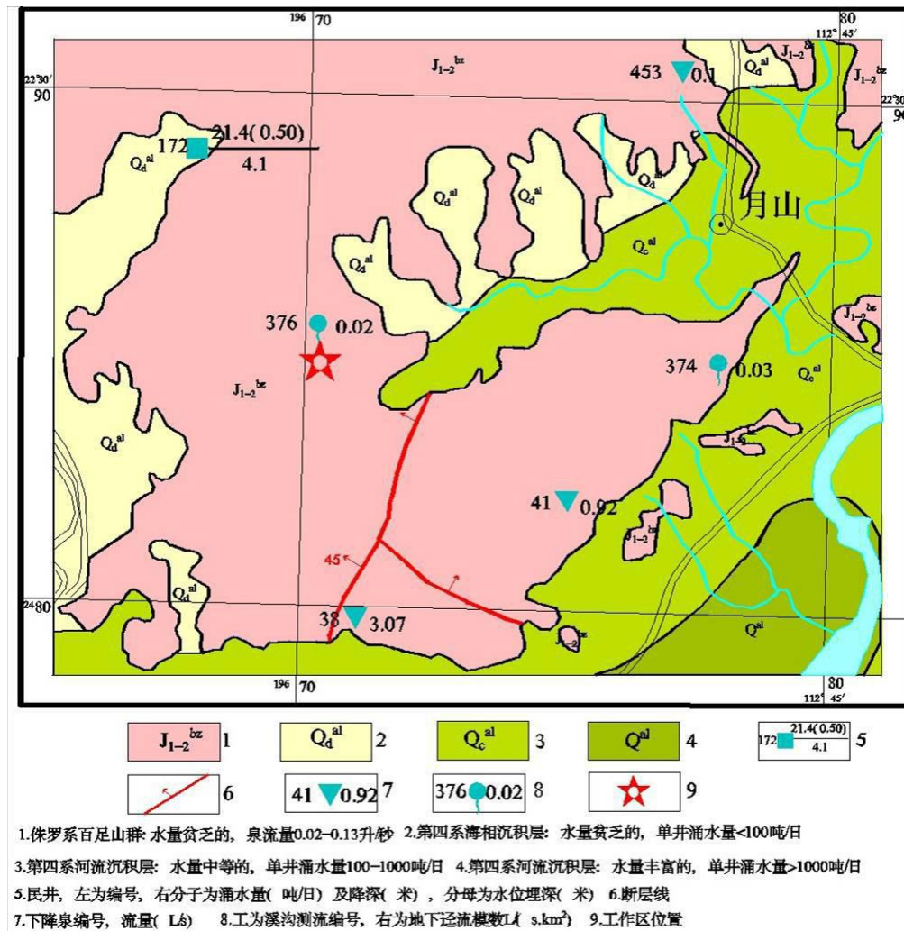
图 4.1-2 项目所在区域水文地质图 (据 1: 20 万开平幅水文地质图修编)
