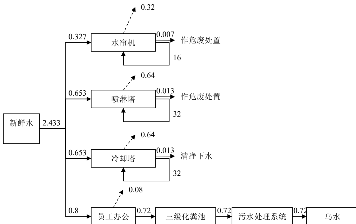
图 3.9-3 项目水平衡图（单位：m 3 /d）
