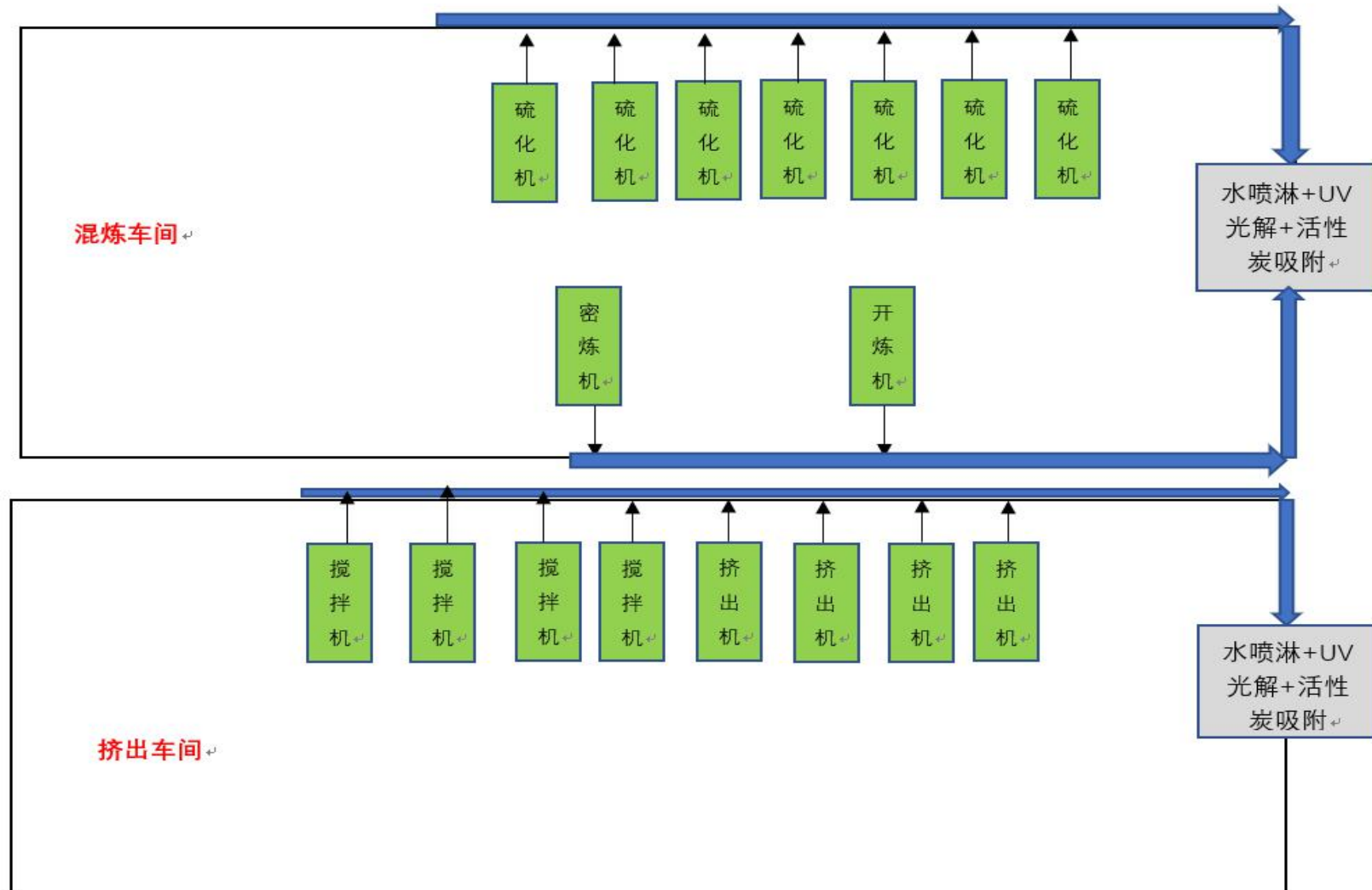
图2.1-5 整改后混炼车间、挤出车间设备布置图
