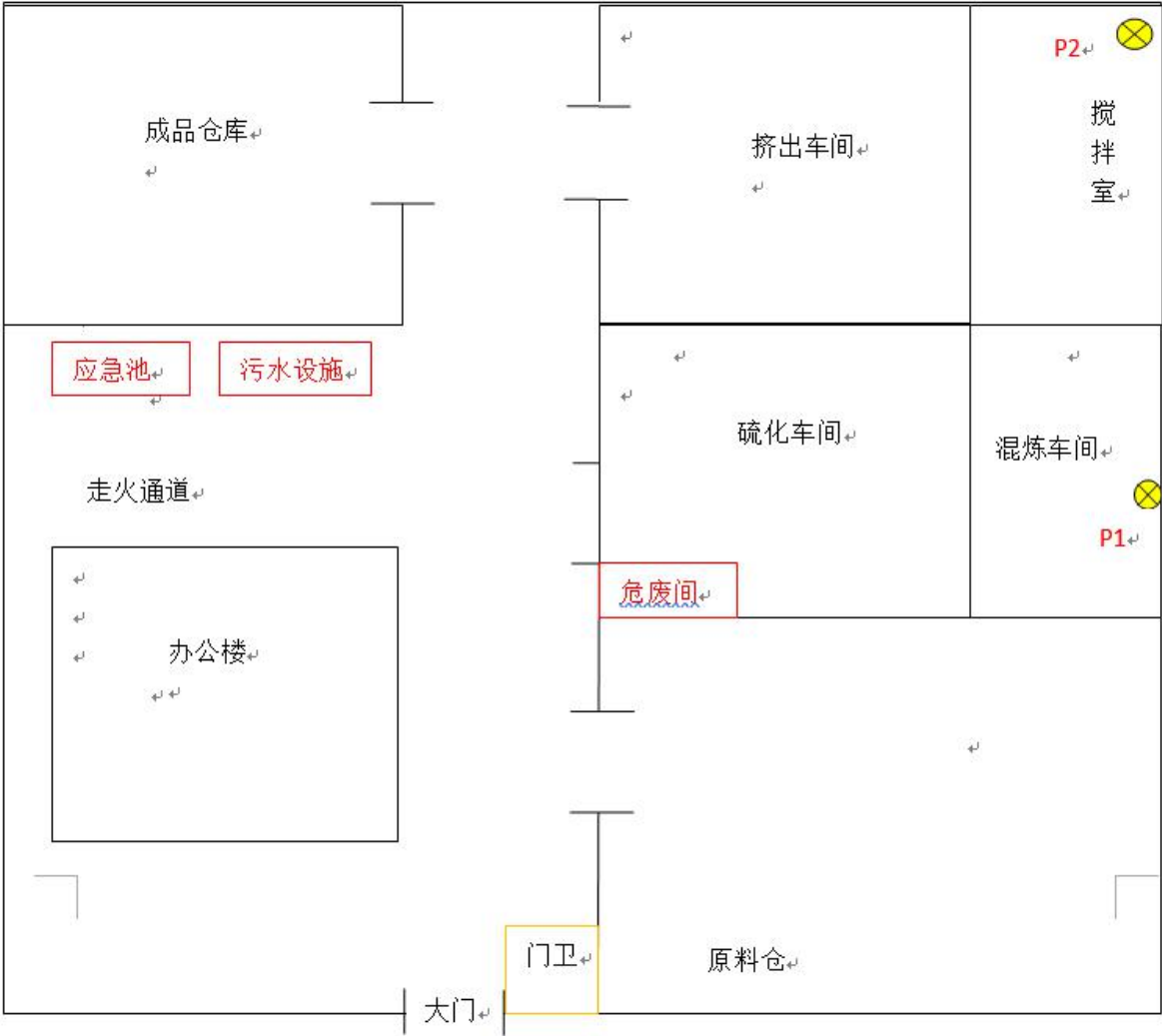
图 2.1-4 整改后总平面布置图
