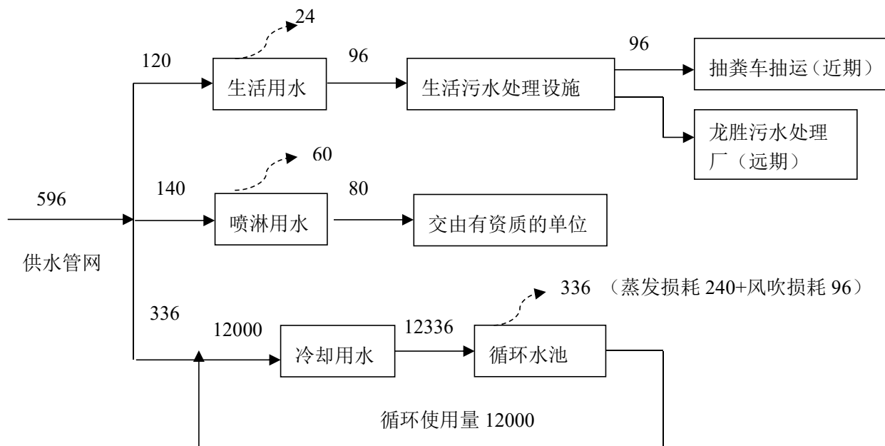
图 2.6-2 项目水平衡图 (单位: \text{m}^3/\text{a} )
