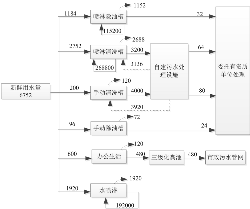
图 5-2 本项目水平衡图（单位：m³/a）
