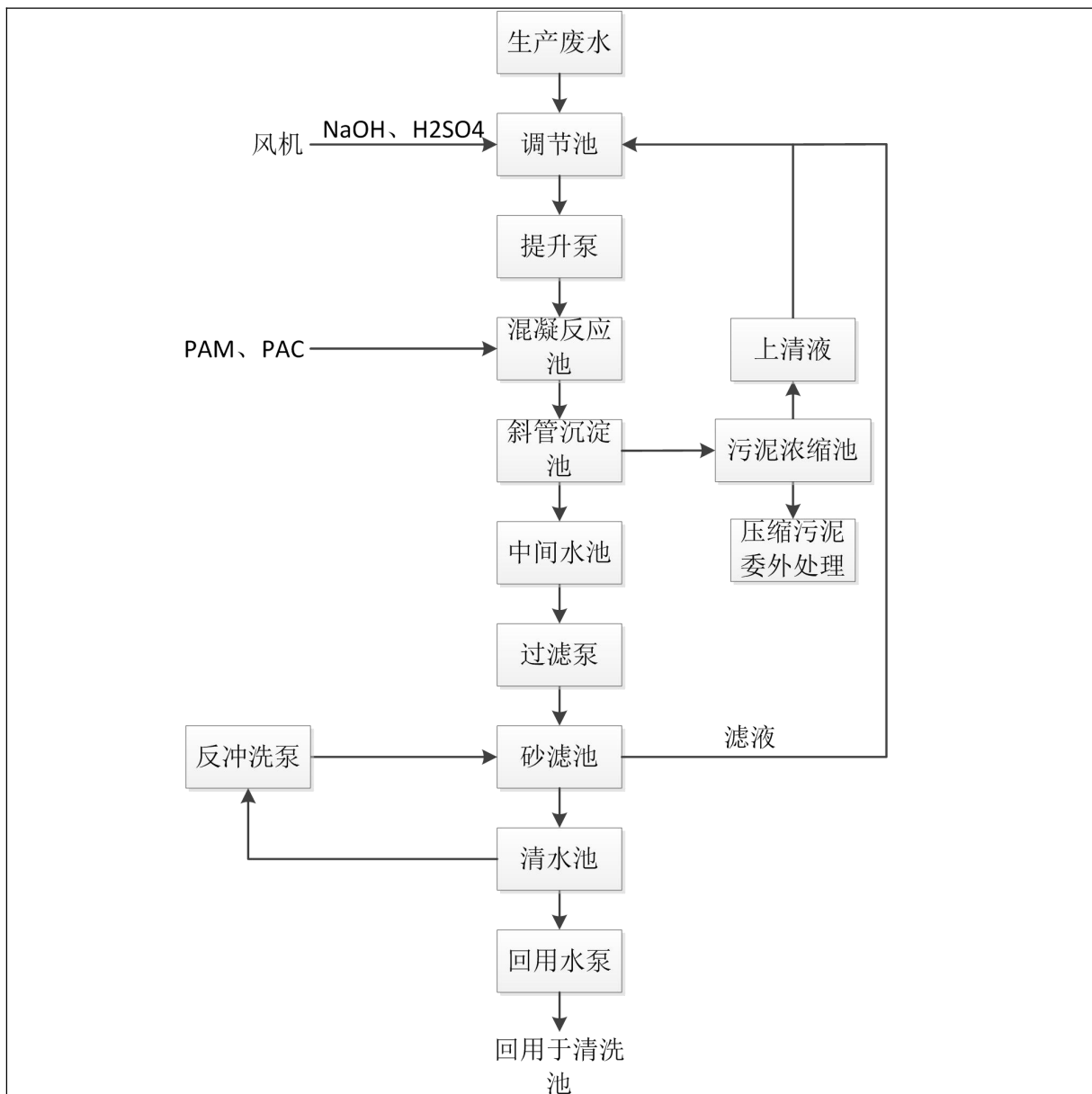
图 7-1 废水处理工艺图
