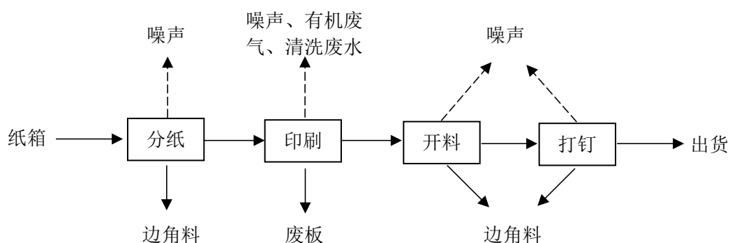
图 5-1 项目工艺流程及产污环节图
