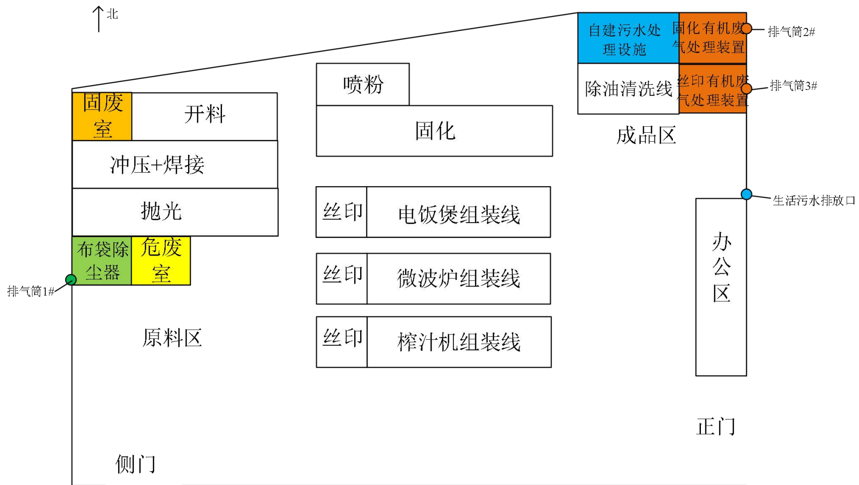
附图 3 项目平面布局图
