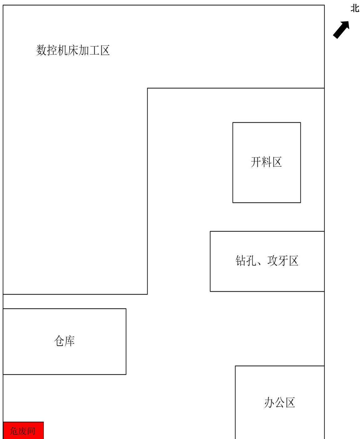
附图 4 厂房平面布置图
