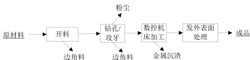
图6-1 项目生产工艺流程图
