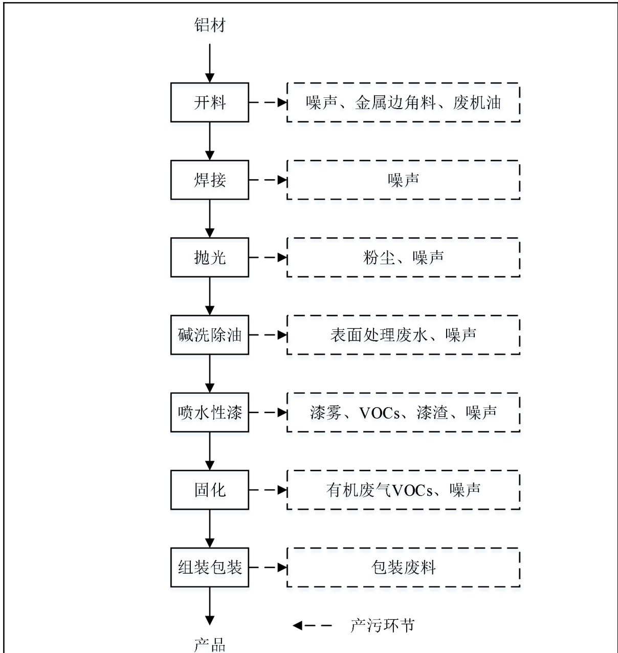
图 5-1 金属摩托车配件生产工艺流程图
