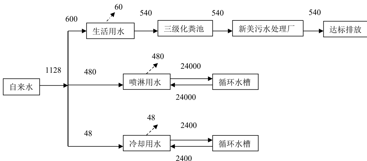
图 5-2 本项目水平衡图 (m³/a)
