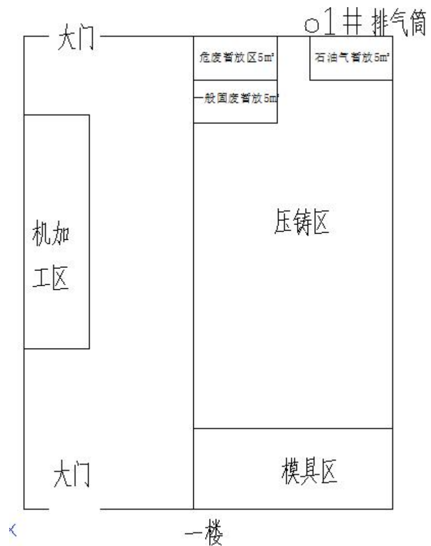
附图 3 项目平面布置图
