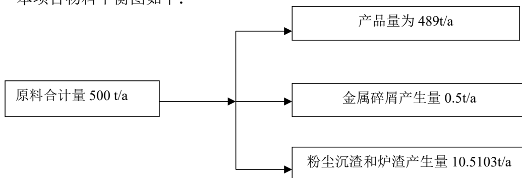
图 1-1 物料平衡图
