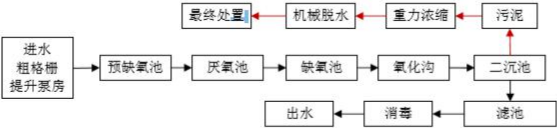
图 7-1 新美污水处理厂污水处理工艺流程图
