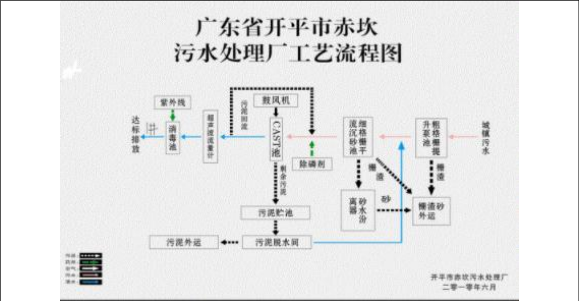
图 4 污水处理工艺流程图
