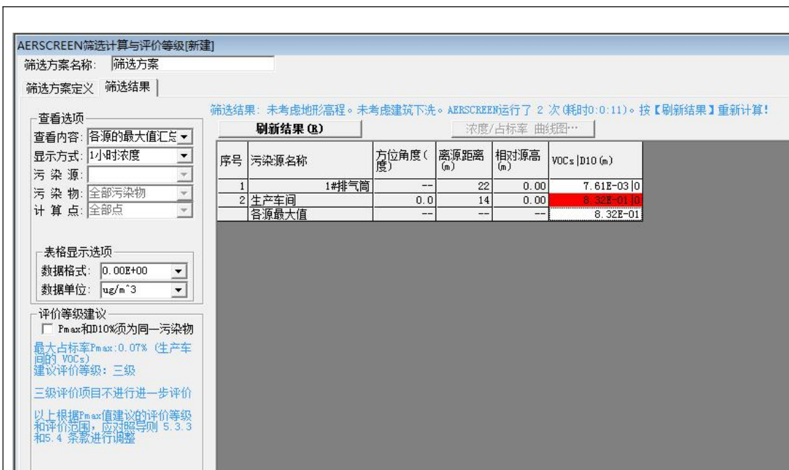
图 2 大气污染物下风向最大质量浓度预测结果截图
