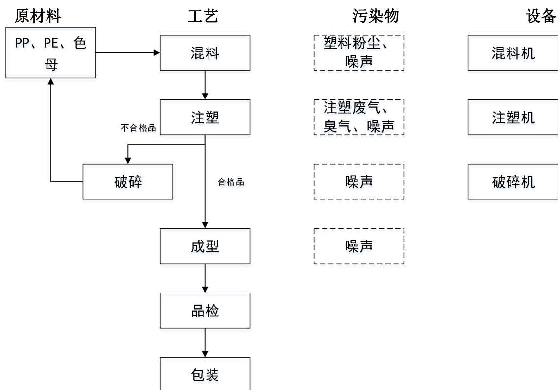
图5-1 项目沙律碗胶盖生产工艺流程图
