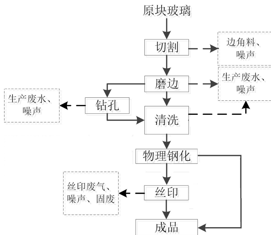
图 5-1 项目工艺流程及产污环节图
