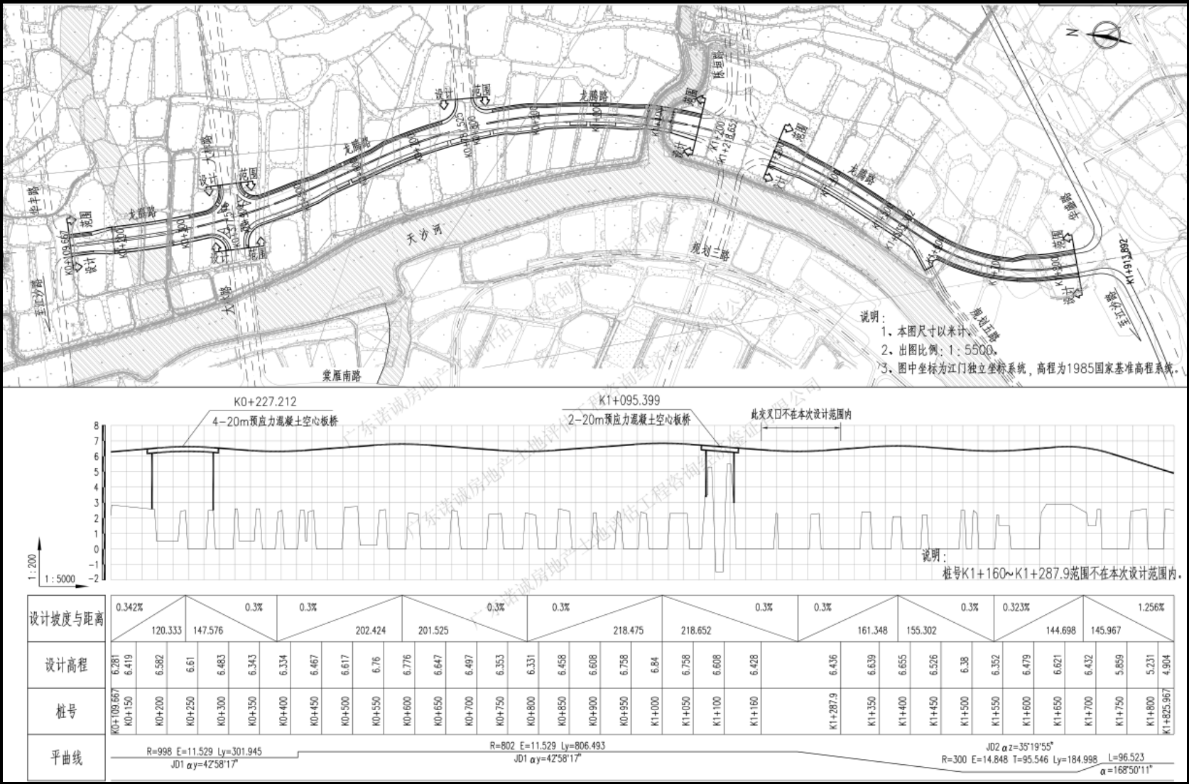
附图二 道路平纵面布置图
