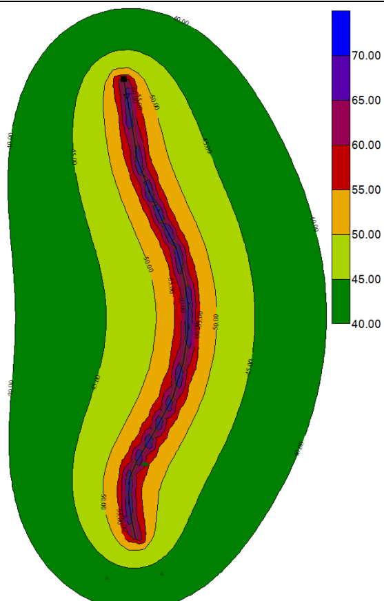
图 7-14 远期昼间噪声预测等声级分布图
