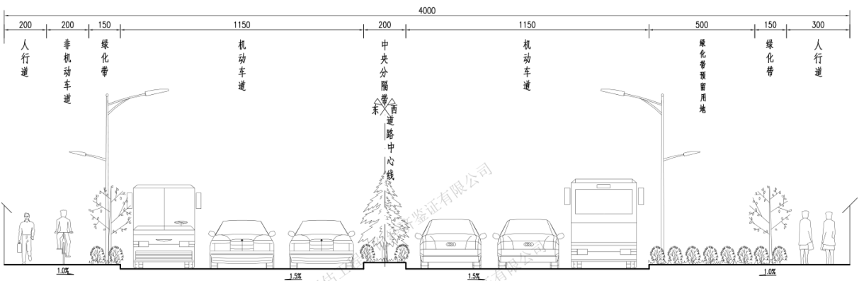
图 1-6 道路标准横断面设计图（二）
