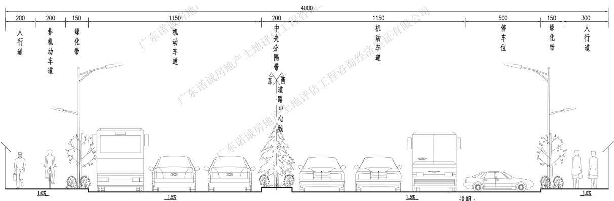
图 1-5 道路标准横断面设计图（一）
