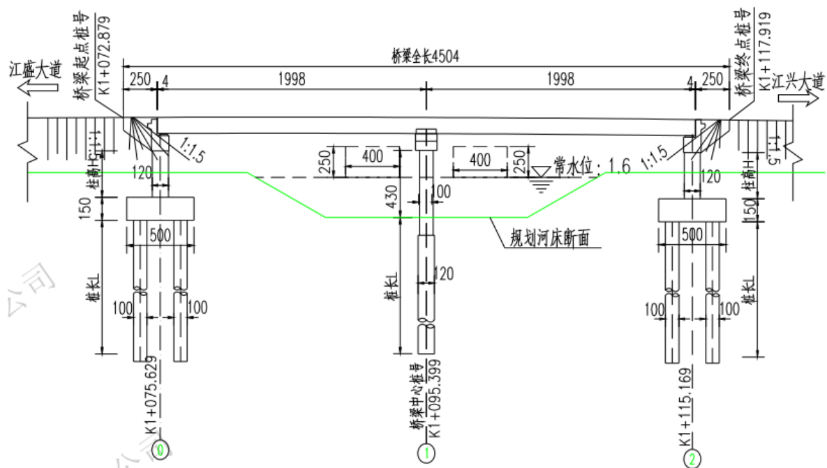
图 1-8 K0+227.212 桥型布置图
