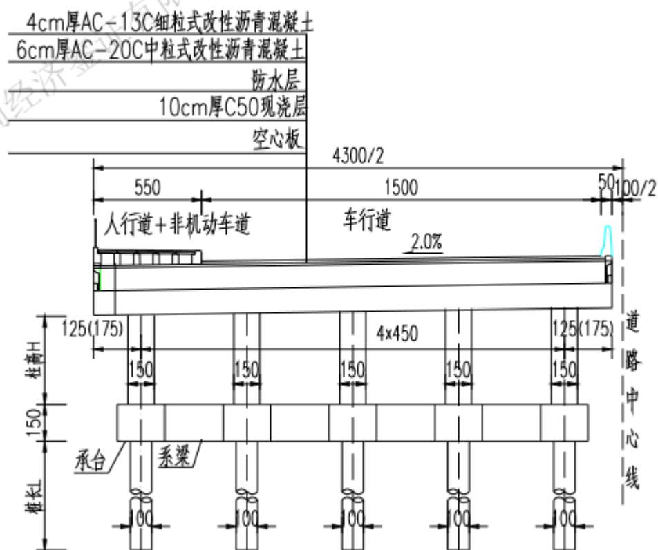
图 1-9 K0+227.212 中桥标准横断面图
