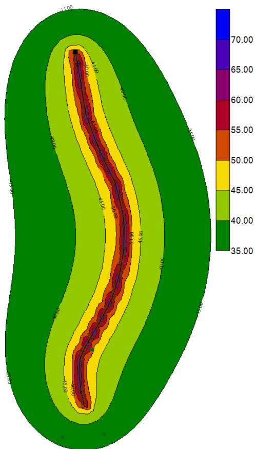
图 7-15 远期夜间噪声预测等声级分布图
