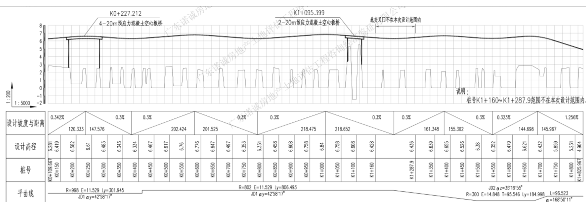
图 1-4 龙腾路设计纵断图
