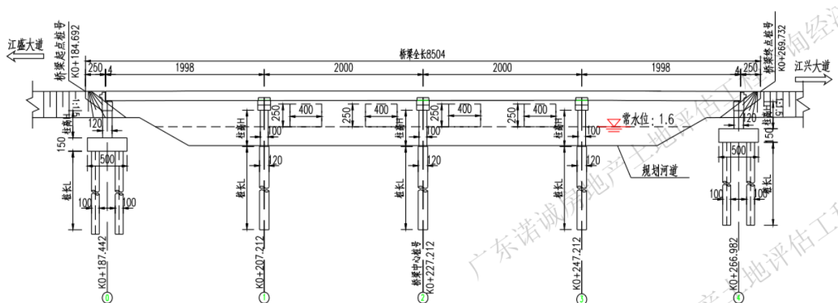
图 1-7 K0+227.212 桥型布置图
