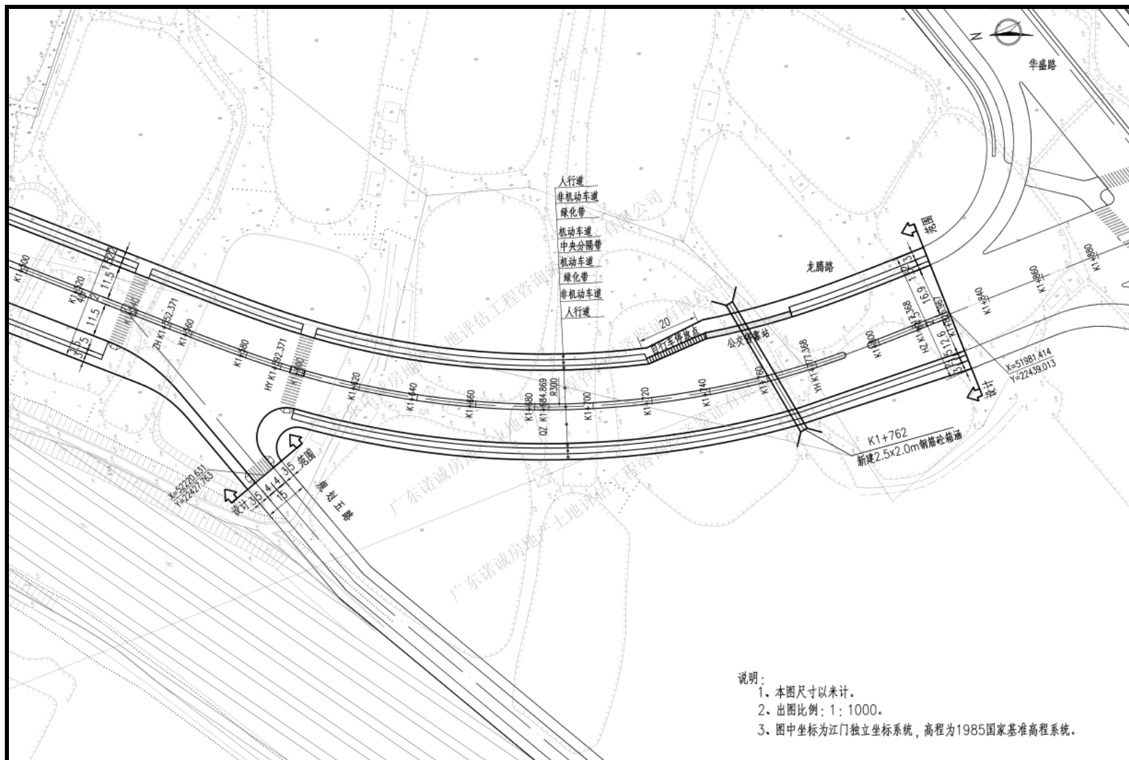
附图三 项目工程平面布局图
