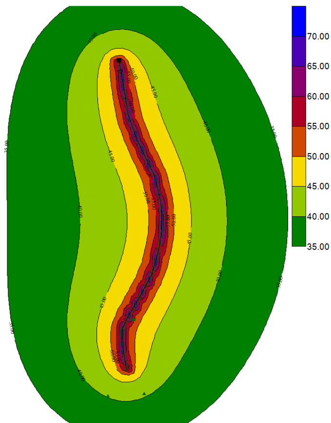
图 7-10 近期昼间噪声预测等声级分布图
