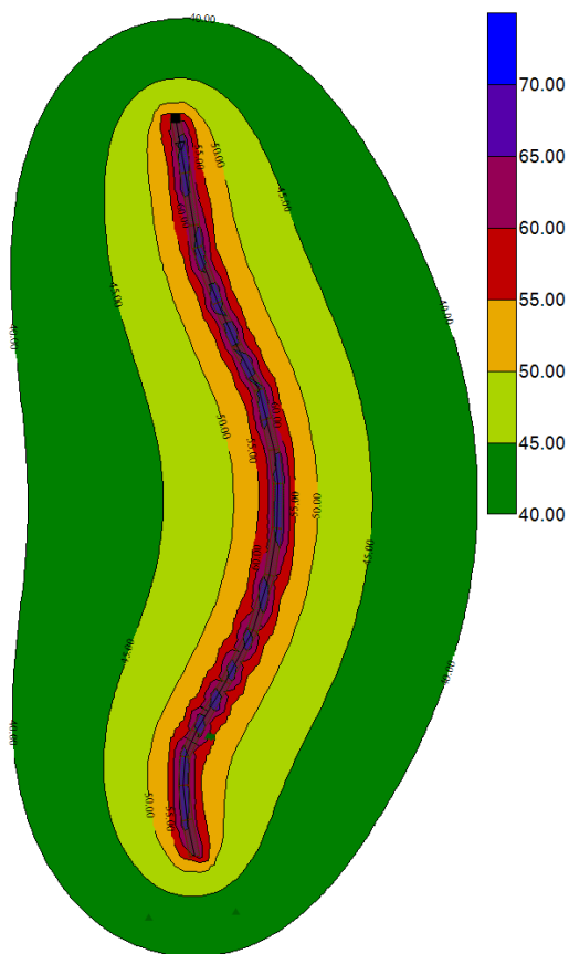
图 7-12 中期昼间噪声预测等声级分布图
