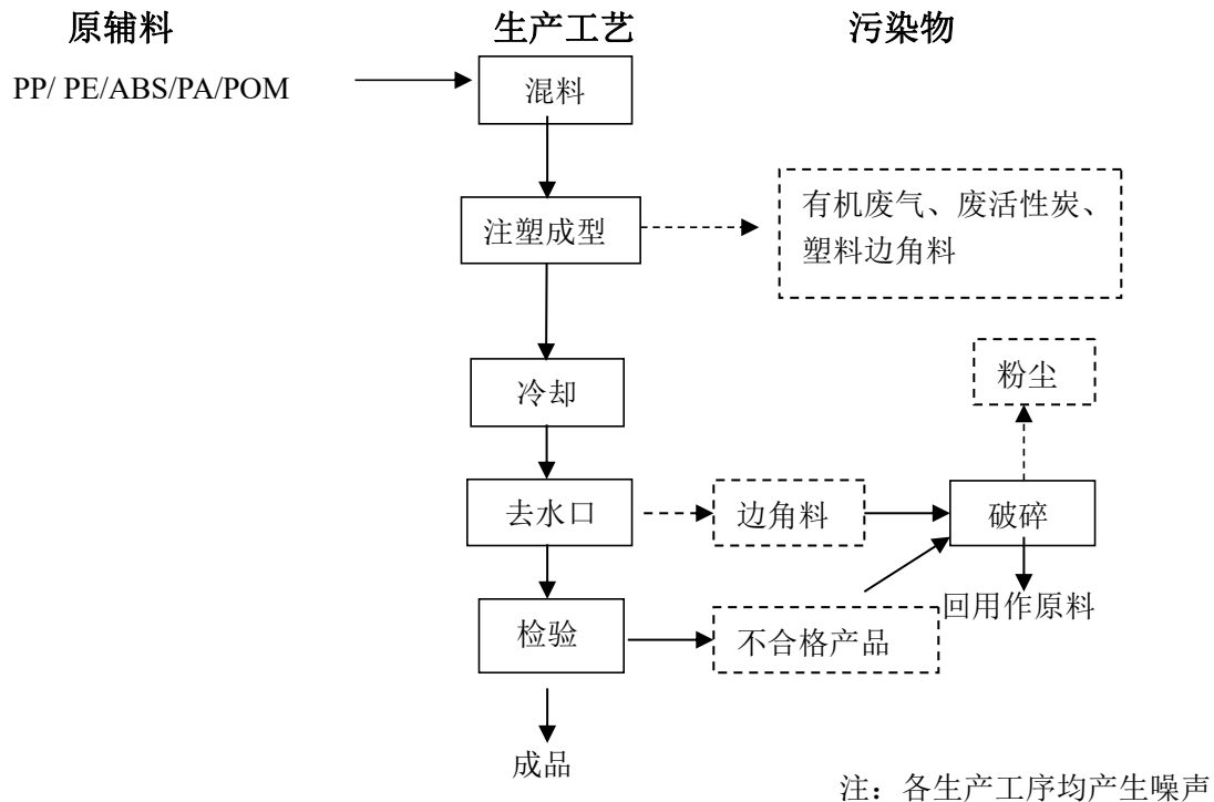
图 5-1 水龙头配件生产工艺流程图
