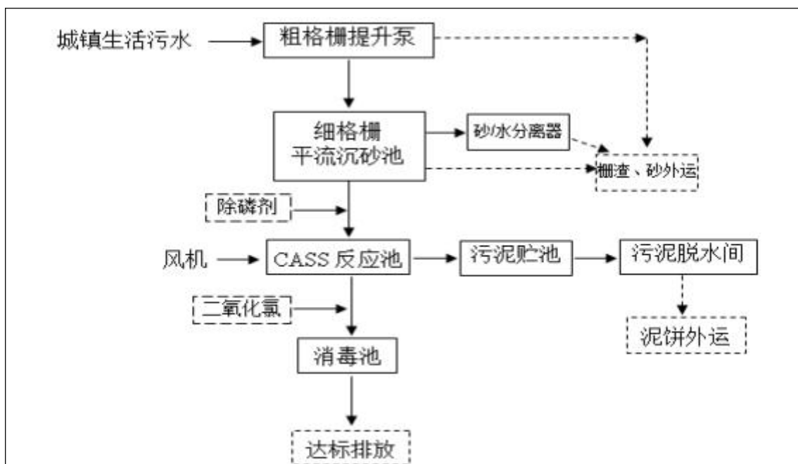
图 7-1 水口镇污水处理厂水处理工艺流程图
