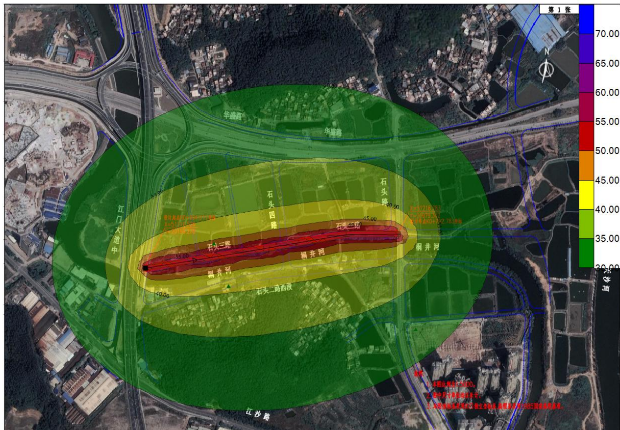
图 7-12 2035 年夜间噪声预测等声级分布图
