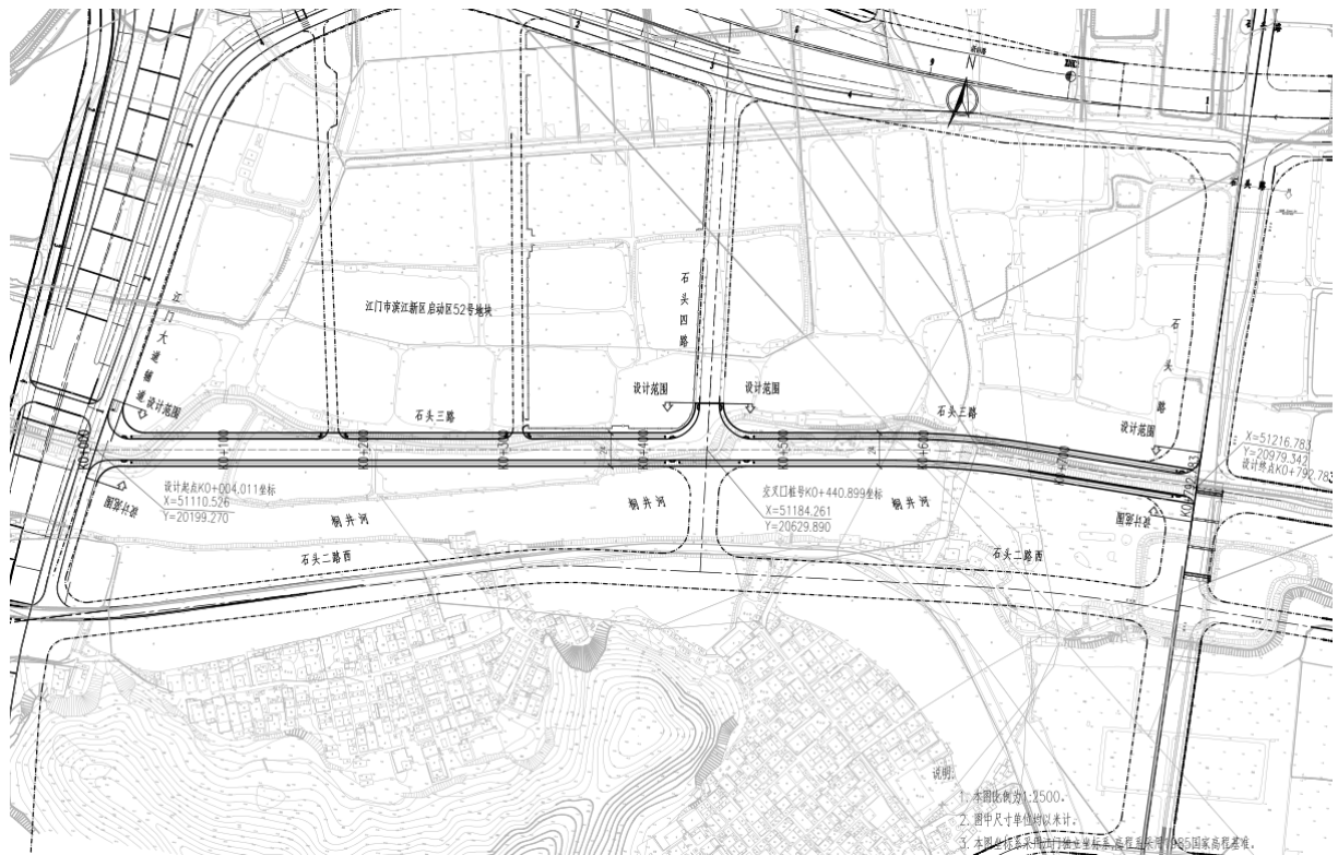
图 1-1 石头三路设计平面图
