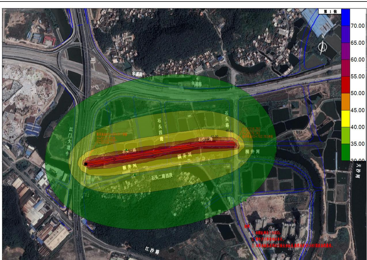
图 7-10 2027 年夜间噪声预测等声级分布图
