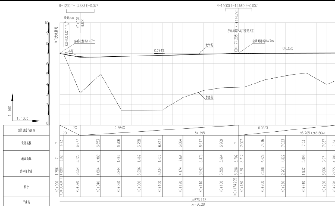
图 1-2 石头三路设计纵断面图
