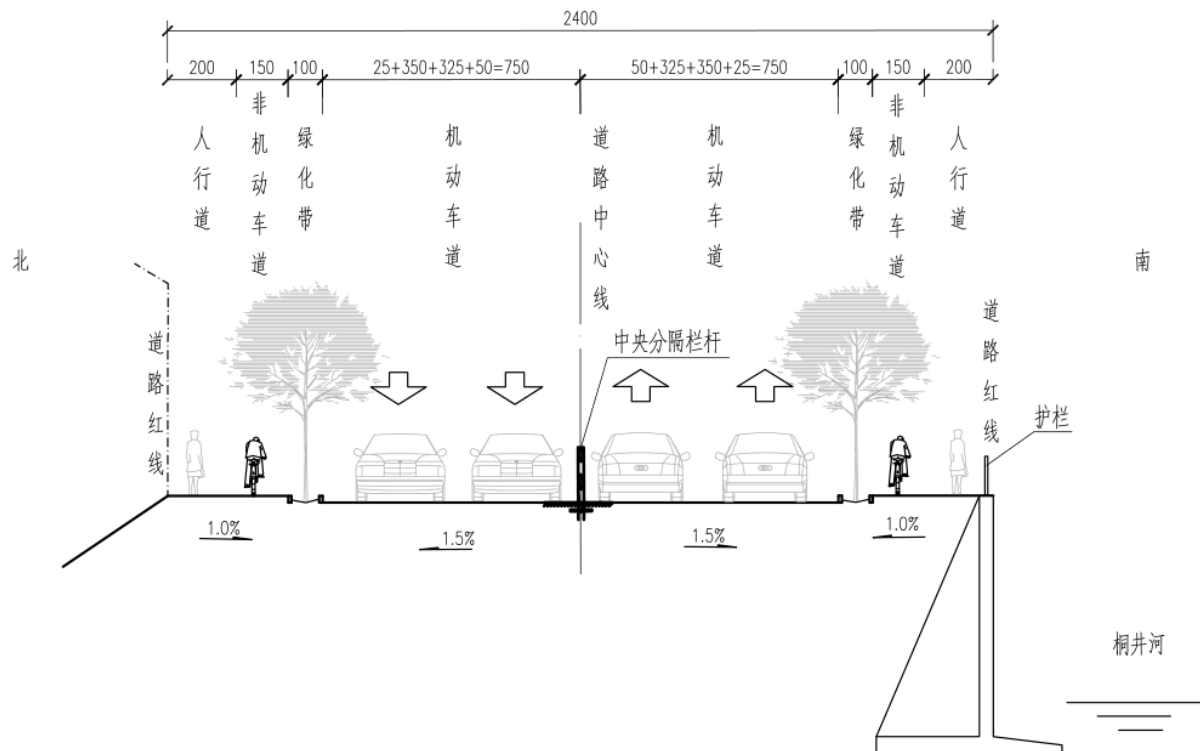
图 1-3 石头路标准横断面设计图（全线）
