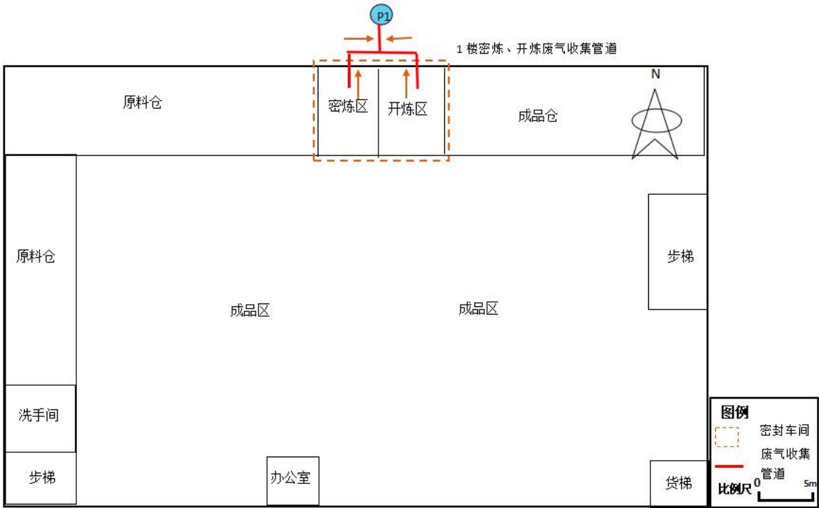
图 9.1-1 一楼密炼、开炼工序废气收集走向图
