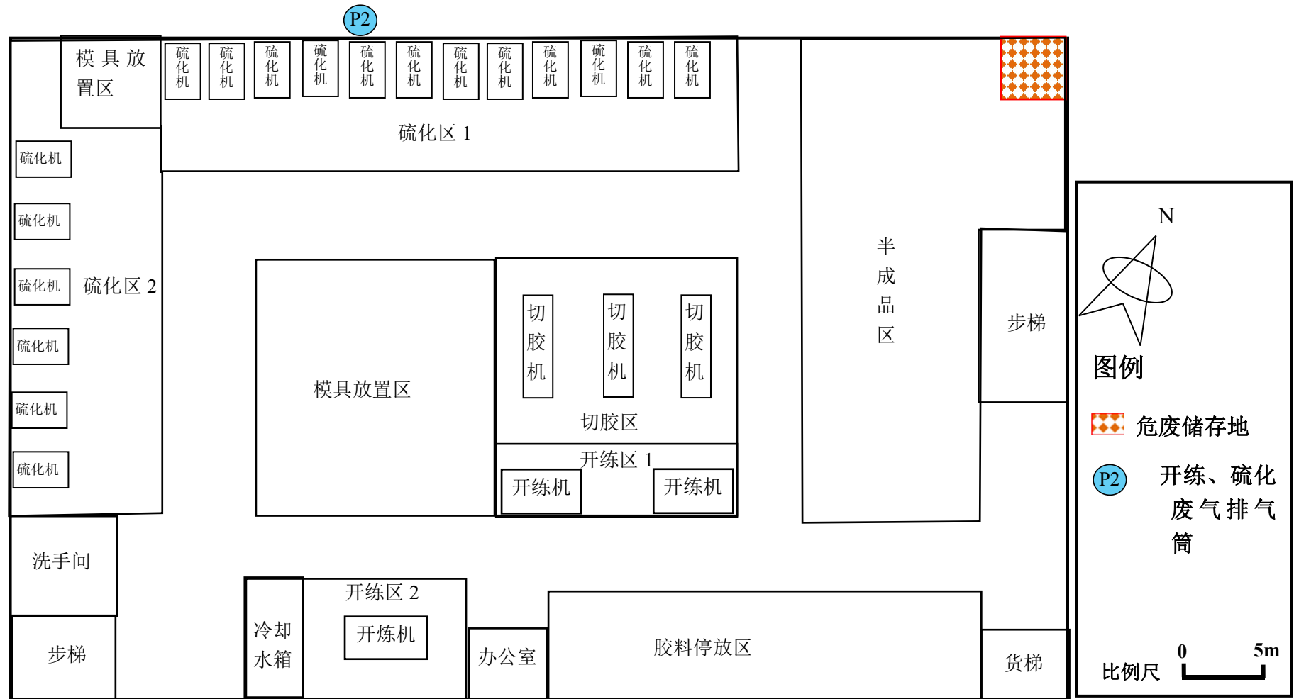
图 3.1-3 厂房第 3 层平面布置图
