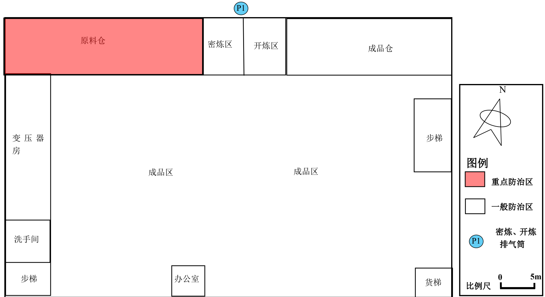
图 8.5-1 厂房第 1 层地下水分区防治示意图
