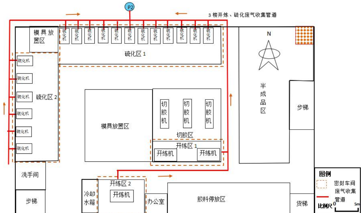
图 9.1-3 三楼开炼、硫化工序废气收集走向图
