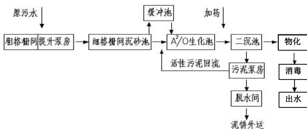
图 8.2-2 A 2 /O 氧化沟流程简图
