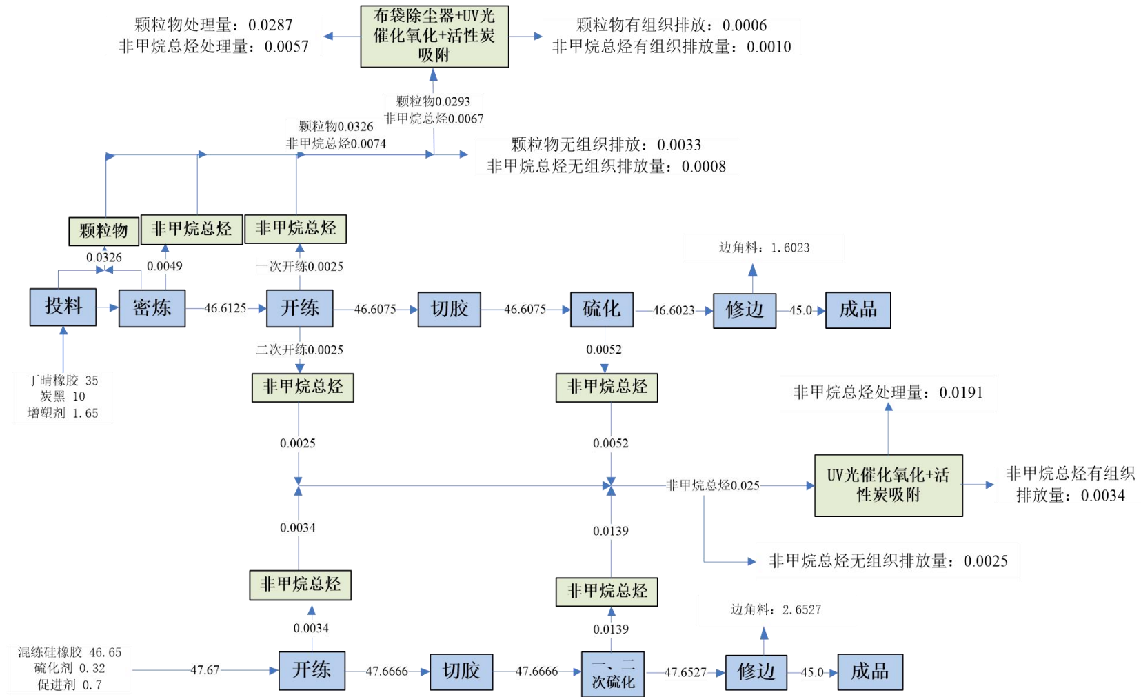
图 3.3-3 项目物料平衡图
