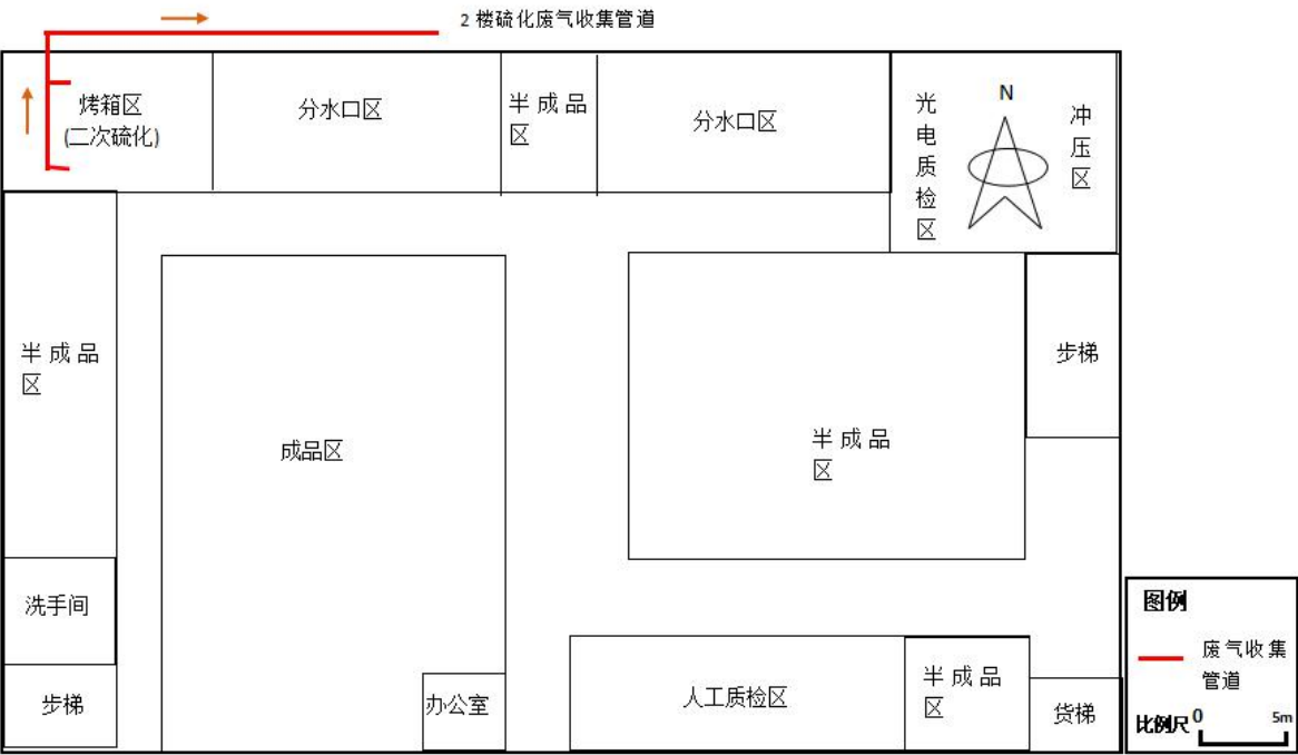
图 9.1-2 二楼硫化工序废气收集走向图
