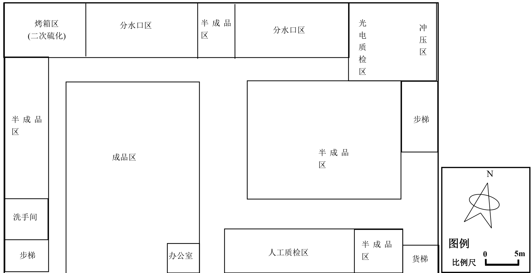
图 3.1-3 厂房第 2 层平面布置图
