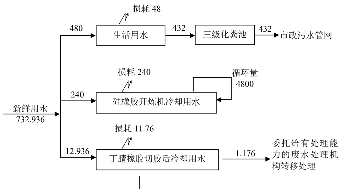
图 3.2-1 项目给排水平衡图 (单位: t/a)
