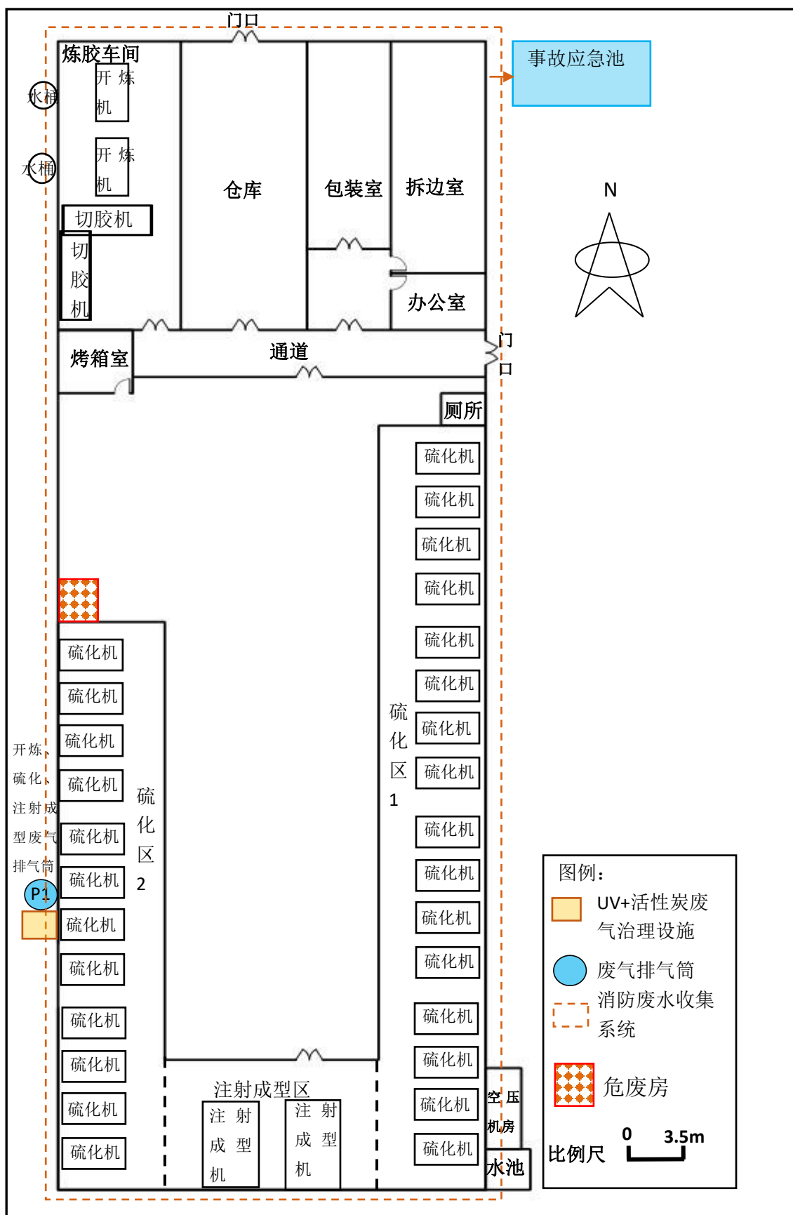
图 3.1-3 项目总平面布置图
