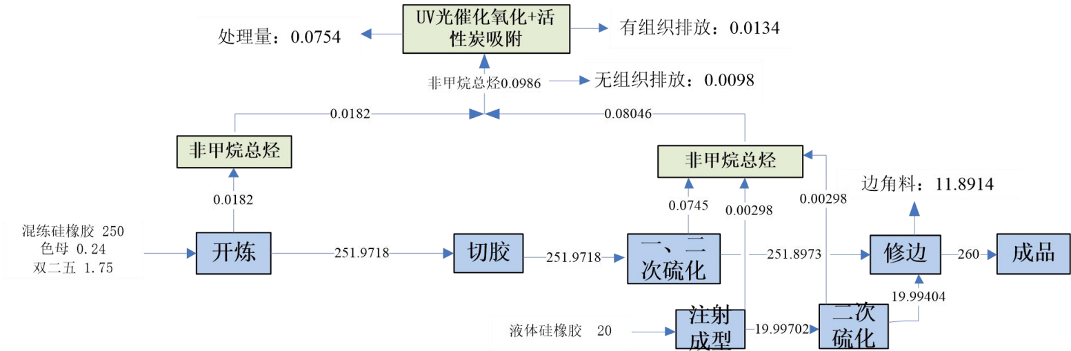
图 3.3-3 项目物料平衡图
