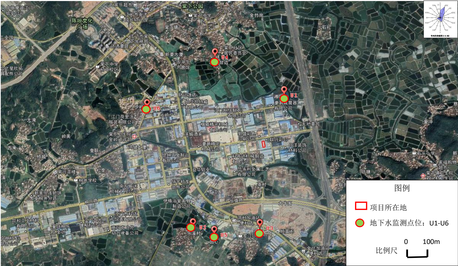
图 5.1-2 项目地下水监测点位图
