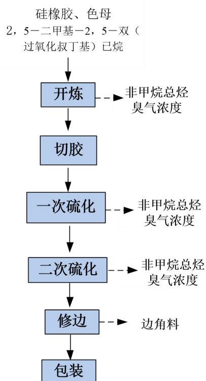
图 3.3-1 项目硅胶制品生产工艺流程图
