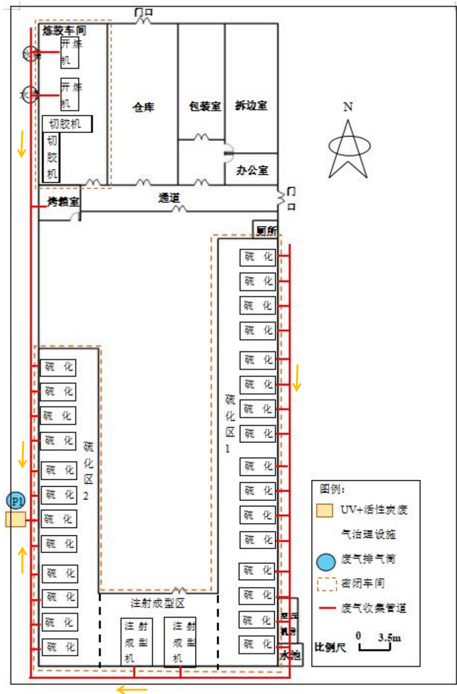
图 9.1-1 开炼、硫化、注射成型工序废气收集走向图
