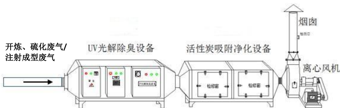
图 9.1-1 有机废气处理流程图
