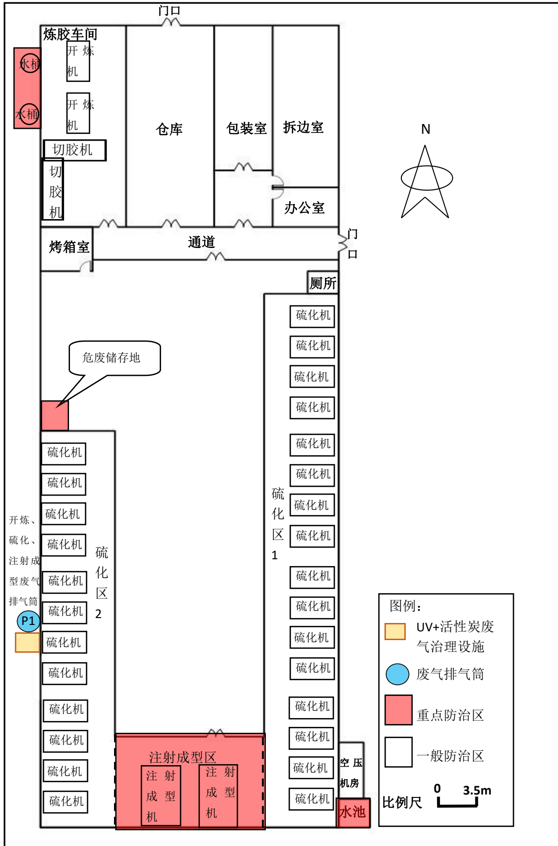
图 8.5-1 地下水分区防治示意图
