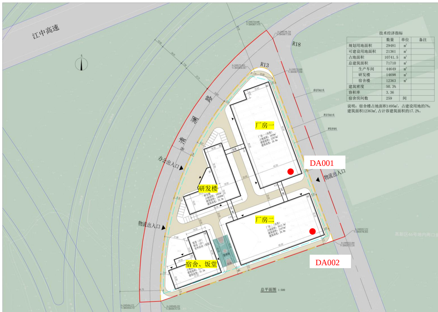
附图 4 项目厂区平面布置图
