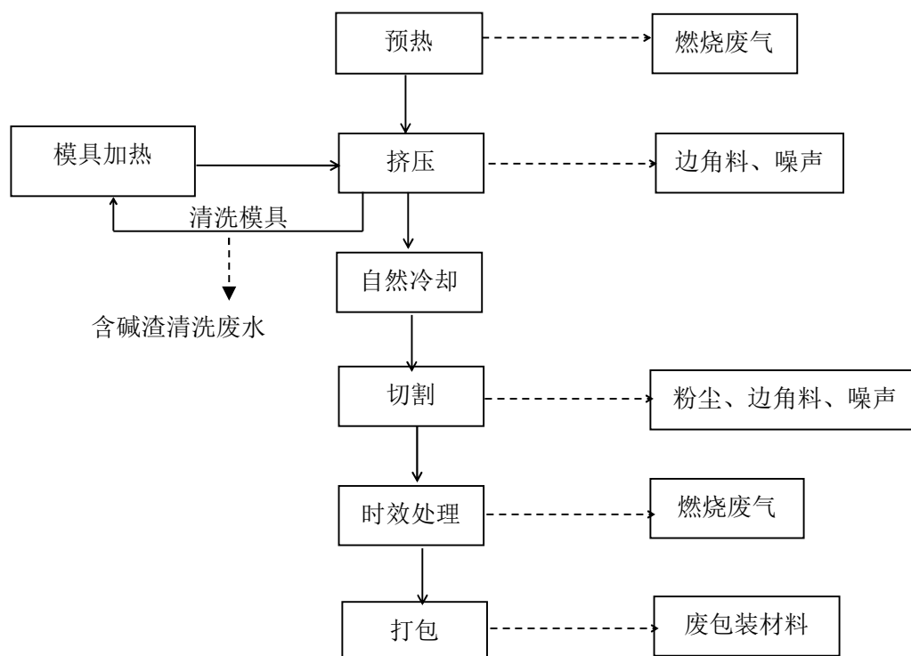
图 6-1 项目生产工艺流程及产污环节示意图
