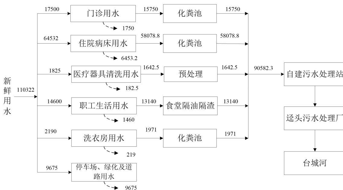
图 1-1 本项目水平衡图（单位：m 3 /a）
