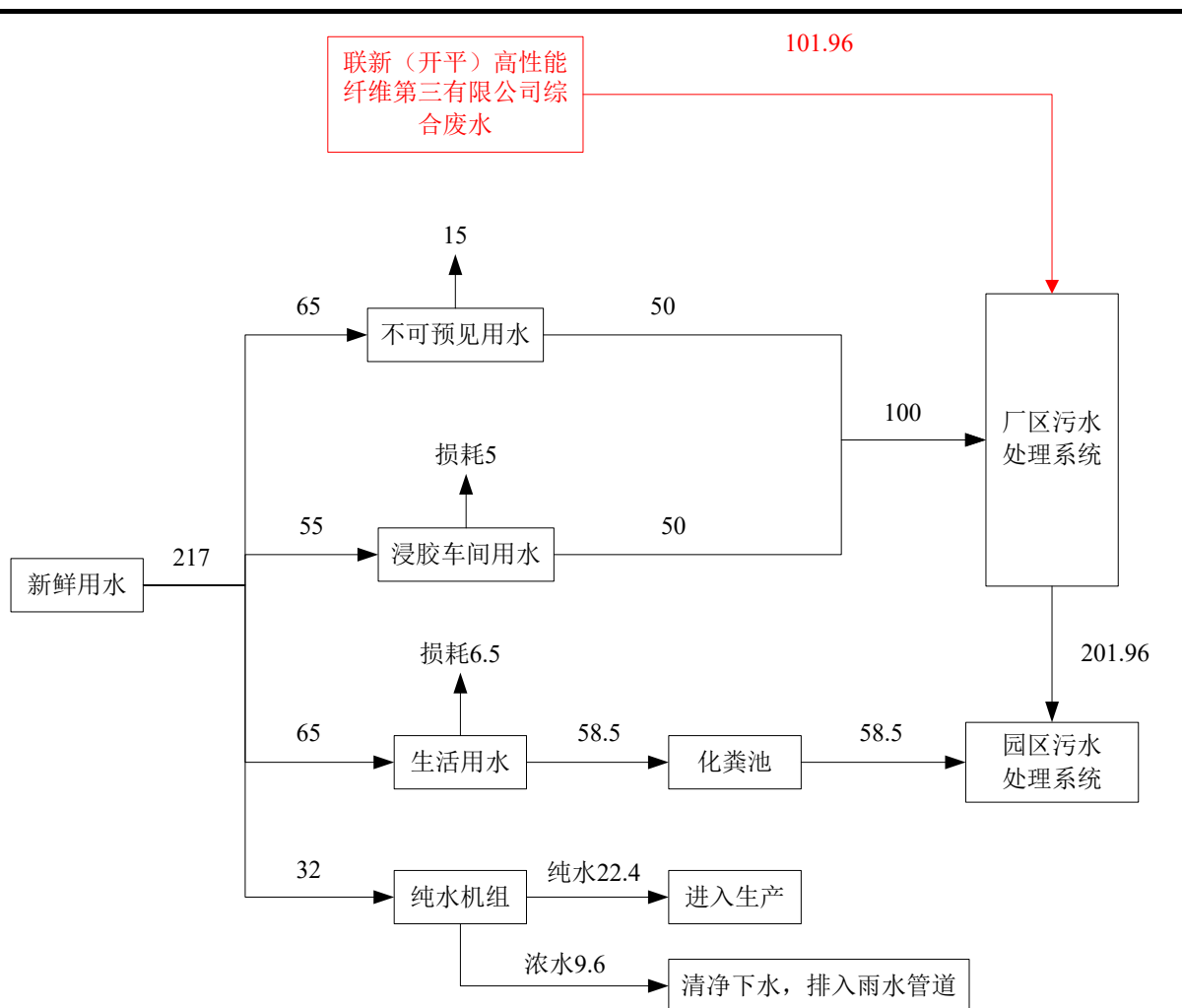
图 1-3 技改前全厂水平衡图（含联新（开平）高性能纤维第三有限公司综合废水） \text{m}^3/\text{d}
