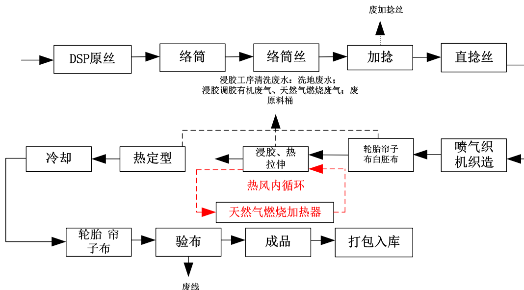
图 1-1 轮胎用帘子布工艺及产排污环节
