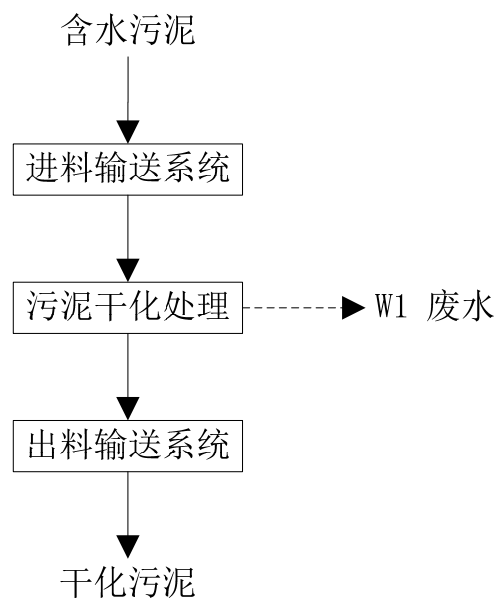
图 5-1 污泥干化工艺流程及产污工序图
