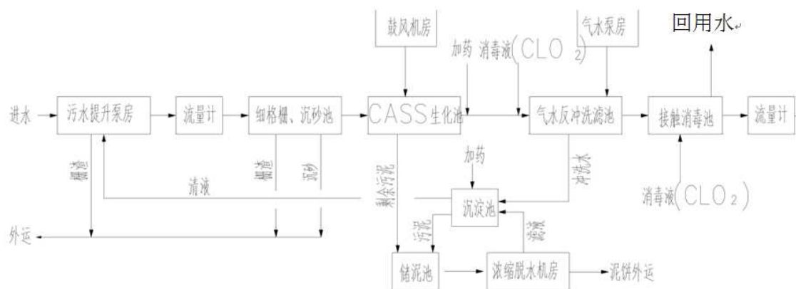
图 7-1 翠山湖污水处理厂拟选工艺流程
