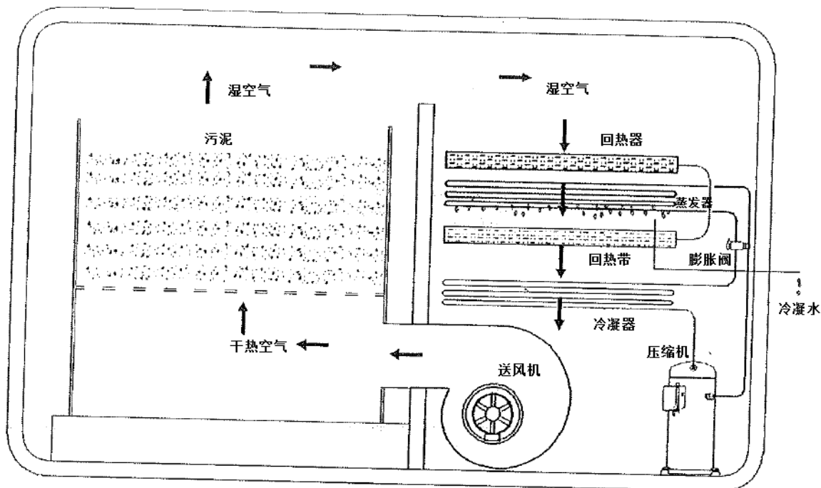
图 5-2 污泥干化机结构示意图
