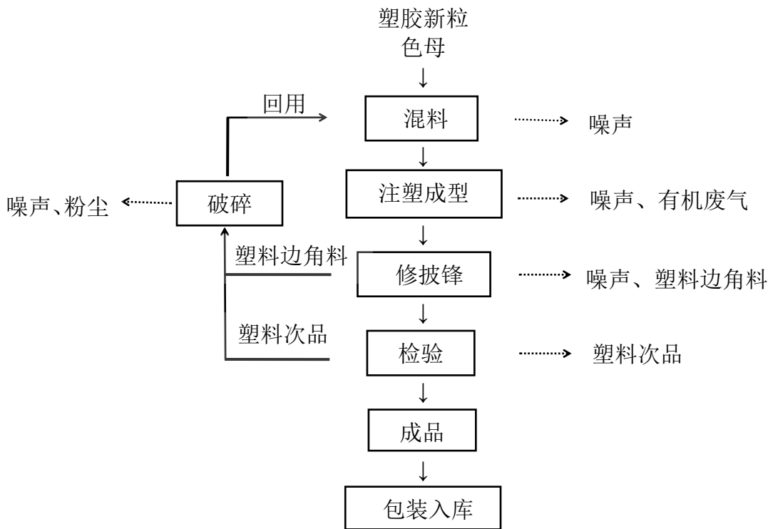
图 5-1 注塑工艺流程图及产污环节
