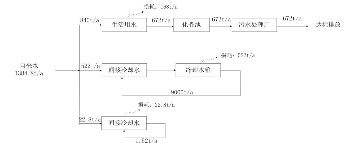
图 3.3-1项目水平衡图
