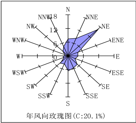
图 4.1-1 开平气象站风向玫瑰图
