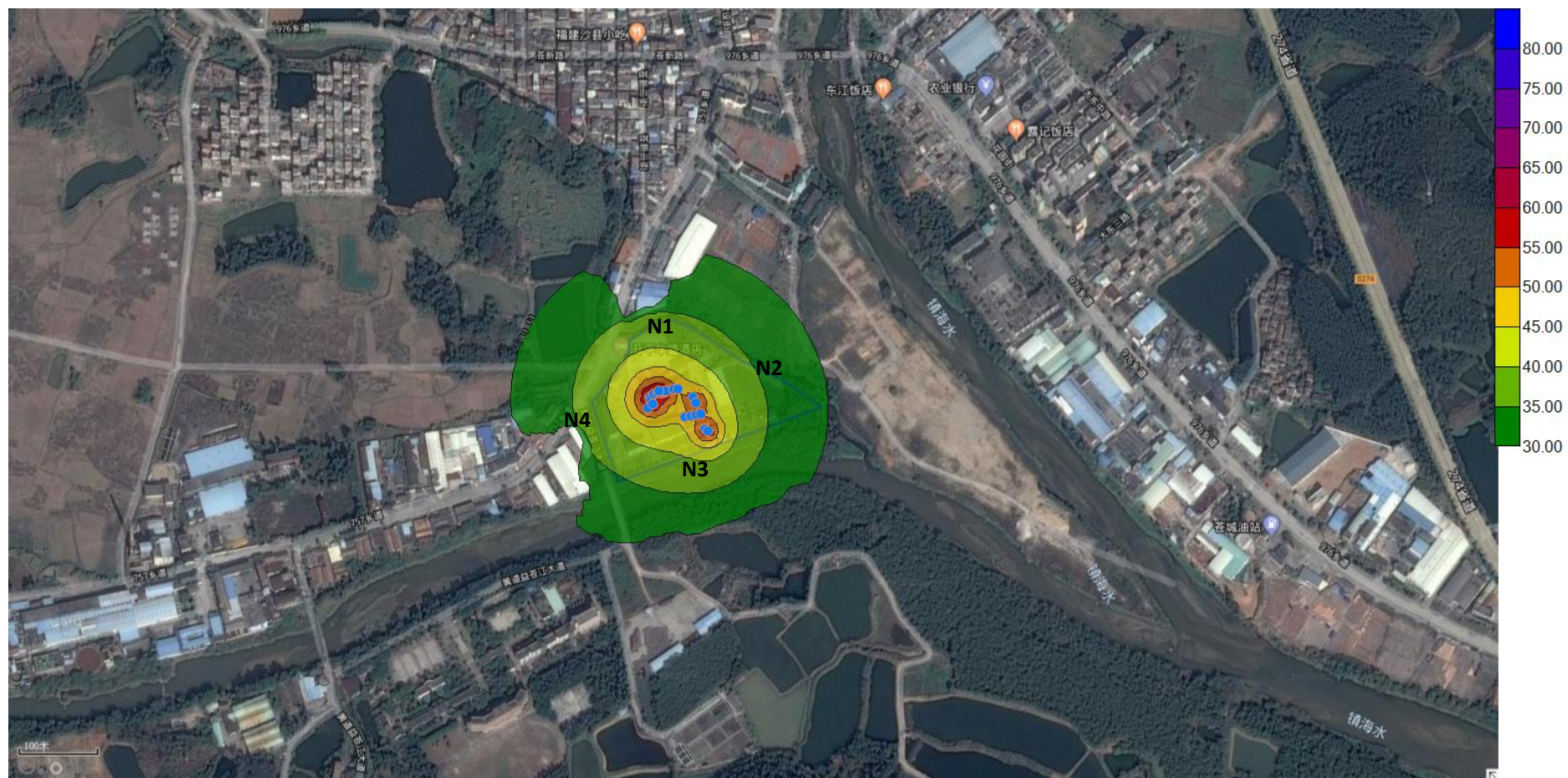
图5.5-1 噪声昼间奉献值线图
