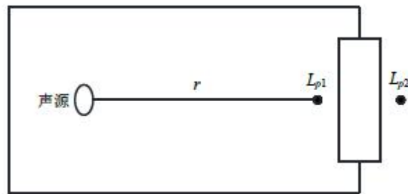
图 7-8 室内声源等效为室外声源图例
