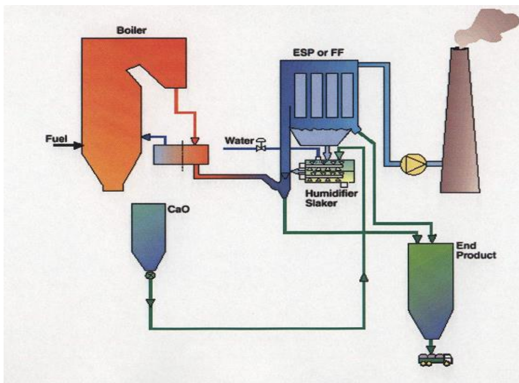
图 8.1-2 烟气 NID 半干法脱硫除尘工艺简图
