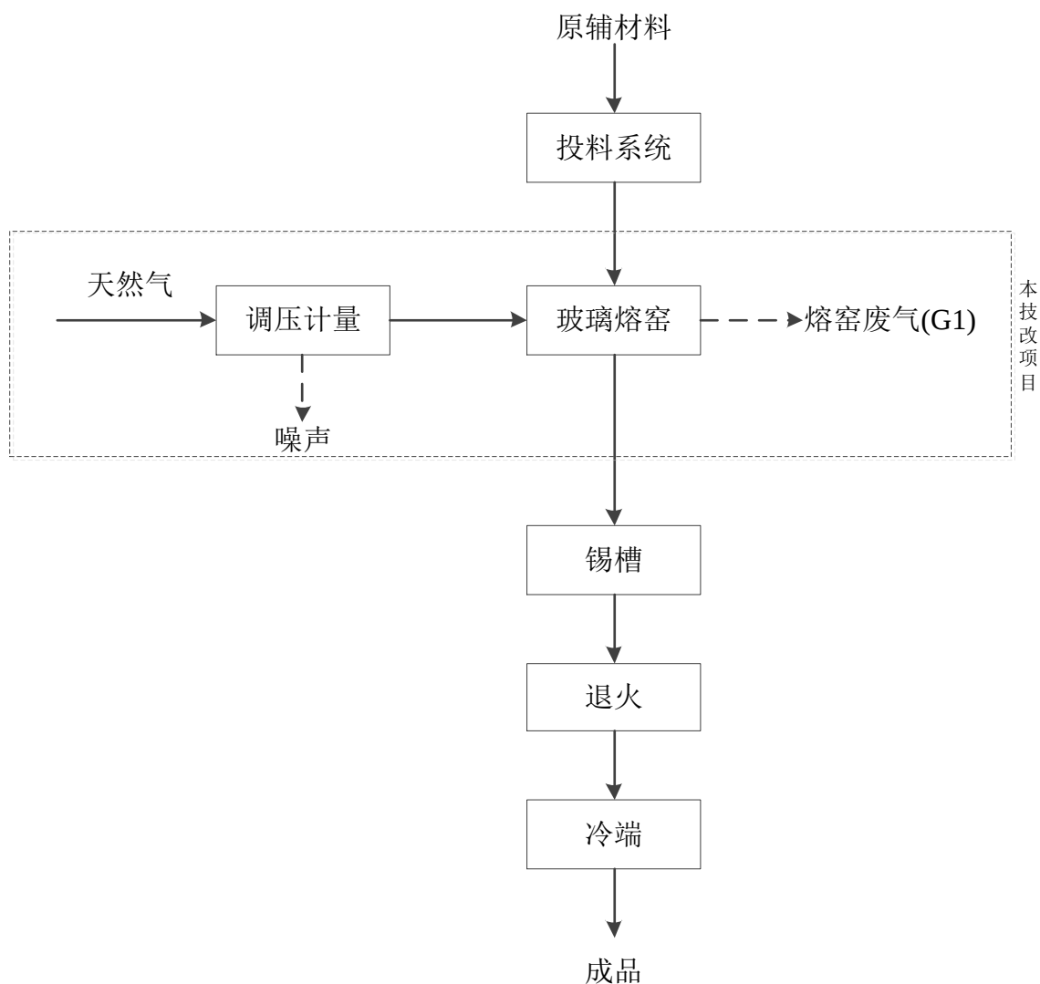
图 4.4-4 技改项目产污环节示意图
