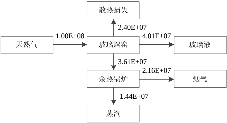
图 4.4-5 技改项目 400t/d 生产线热量平衡图 (KJ/h)
