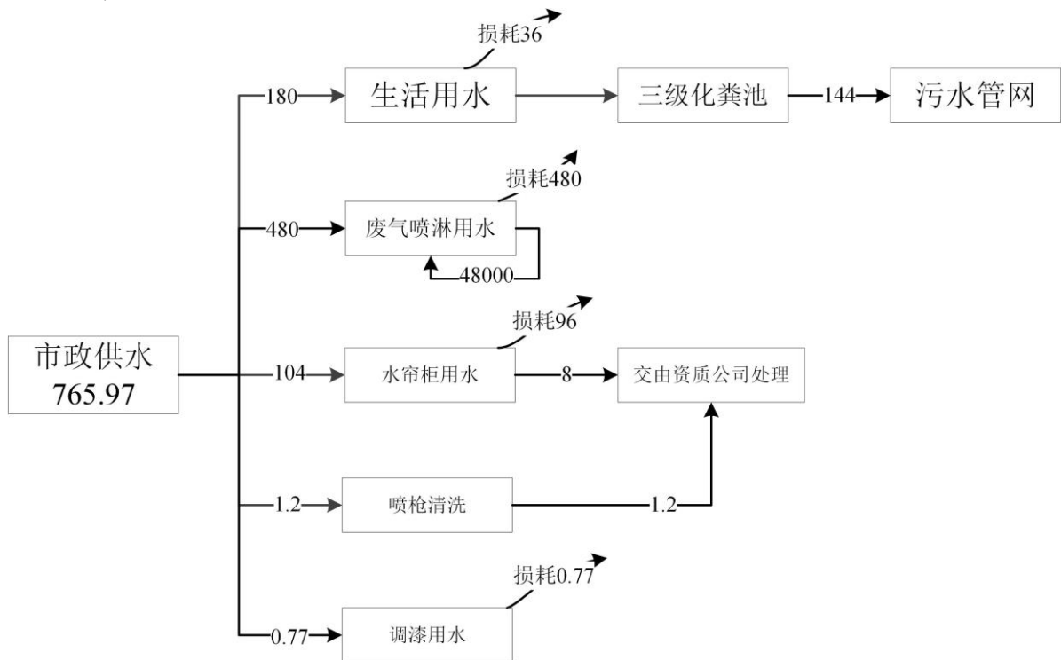
图 1-1 水平衡图 (m 3 /a)
