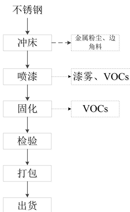
图 5-1 生产工艺流程图
