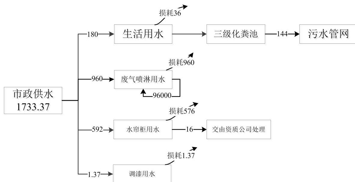
图 1-1 水平衡图 (m 3 /a)
