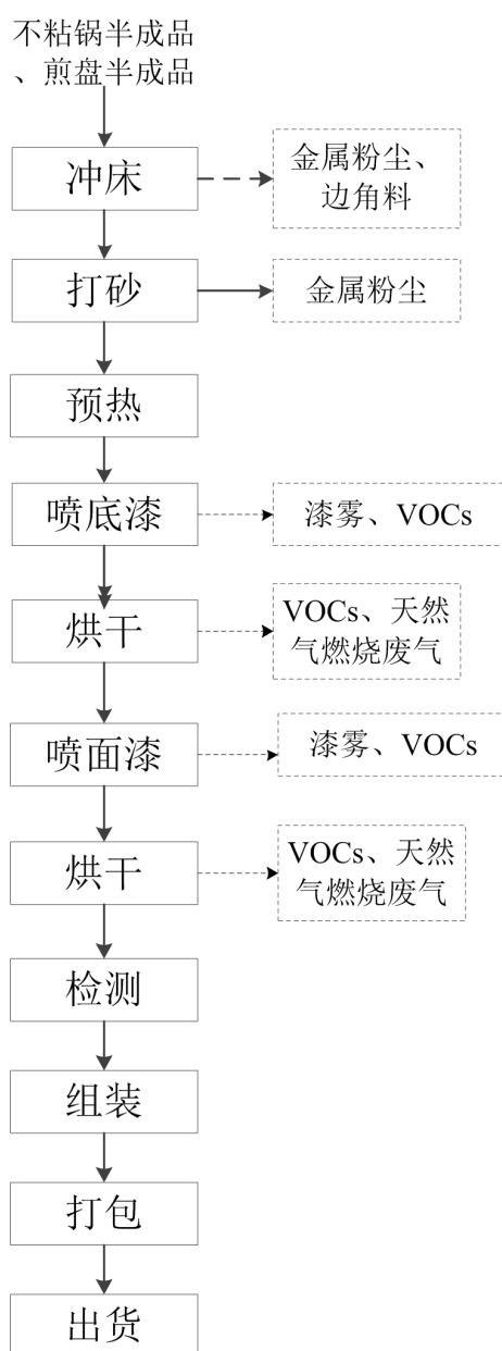
图 5-1 项目工艺流程图
