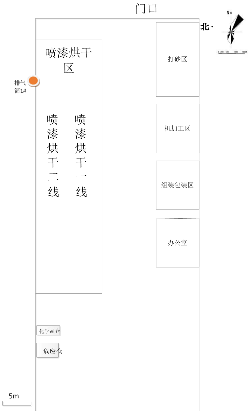
附图 4 项目厂区平面图
