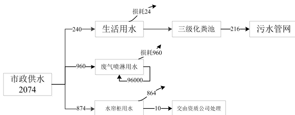
图 1-1 水平衡图
