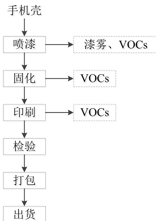
图 5-1 生产工艺流程图
