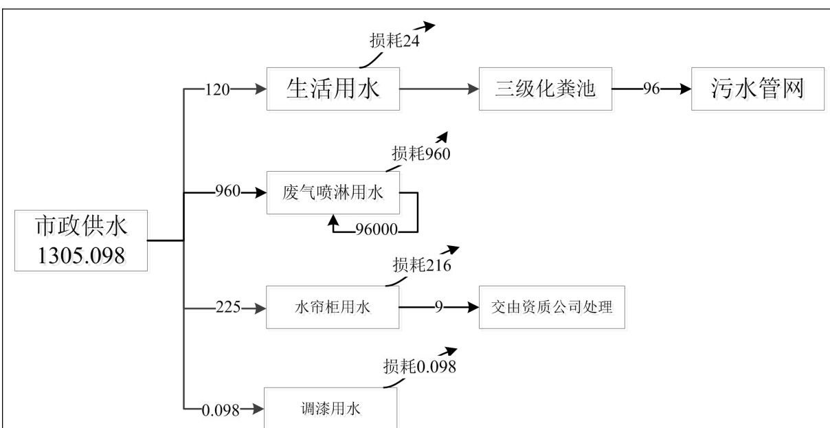
图 1-1 水平衡图 (m³/a)
