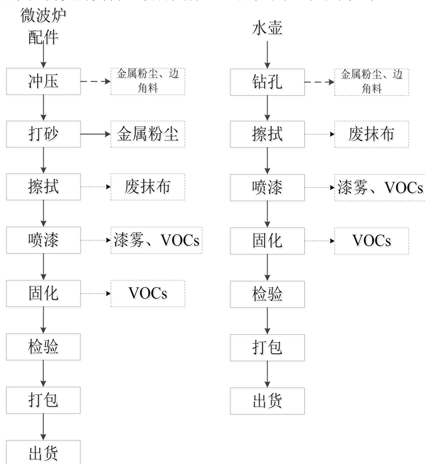
图 5-1 生产工艺流程图
