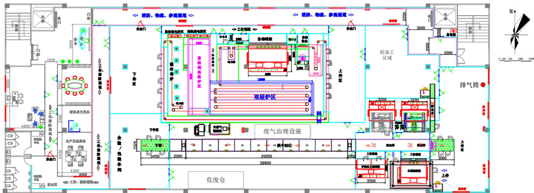
附图 4 项目厂区平面图 (5 楼)
