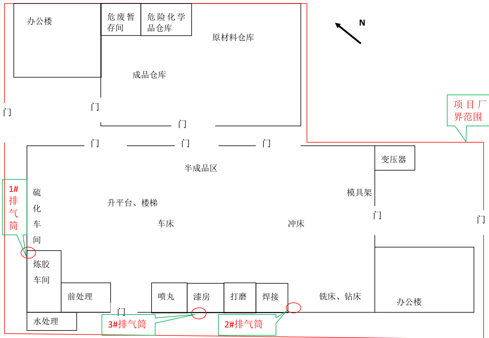
附图 5 项目厂区总平面图
