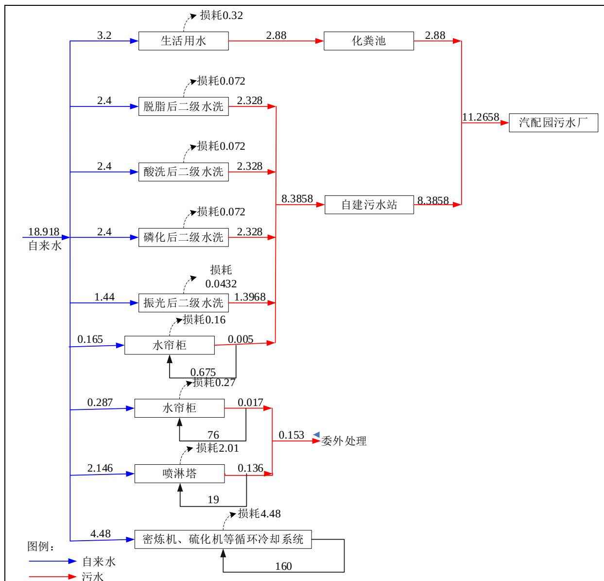
图 1-1 项目水平衡图 (m³/a)
