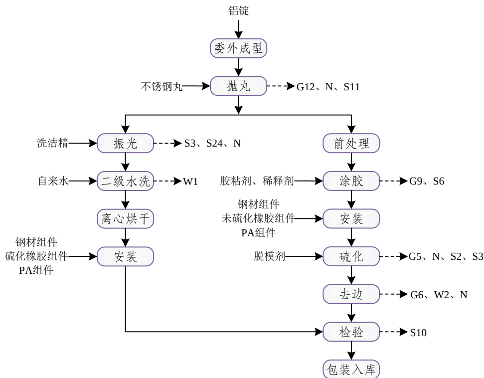
图 5-3 钢材铝材尼龙橡胶类产品生产工艺流程及产污节点图
