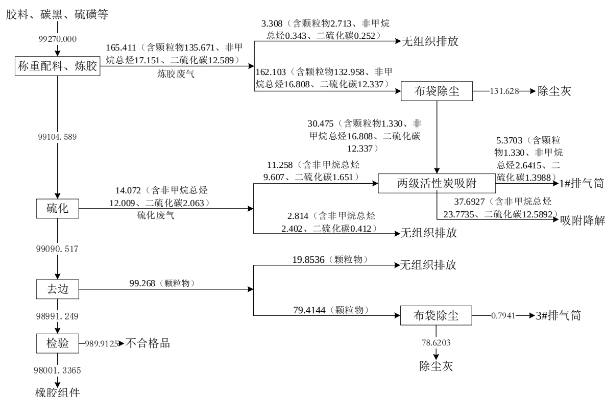
图 5-4 本项目橡胶物料平衡图 (kg/a)
