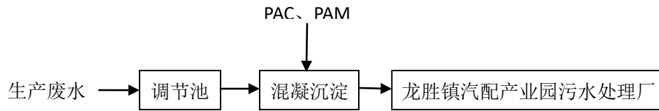
图 7-3 厂内污水站处理工艺流程图
