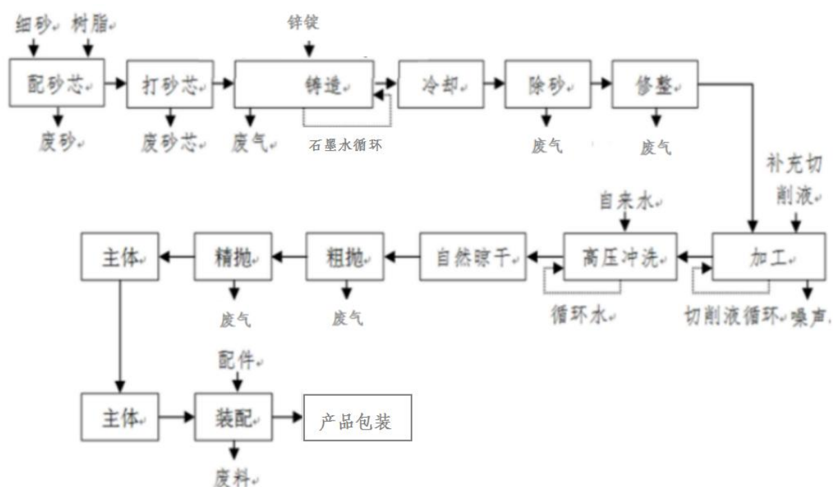
图 5-2 锌质产品生产工艺流程
