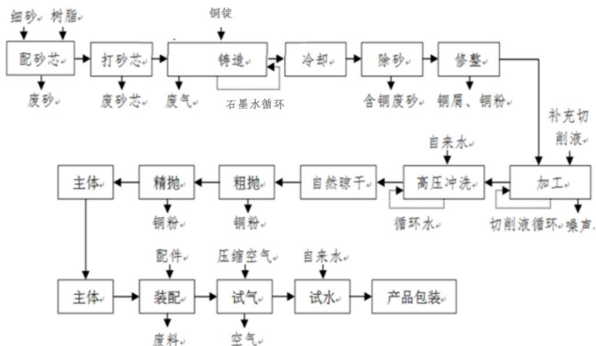
图 5-1 铜质产品生产工艺流程
