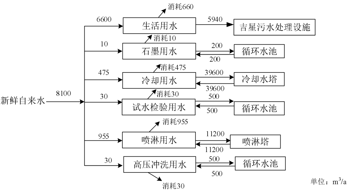
图 5-2 项目水平衡图
