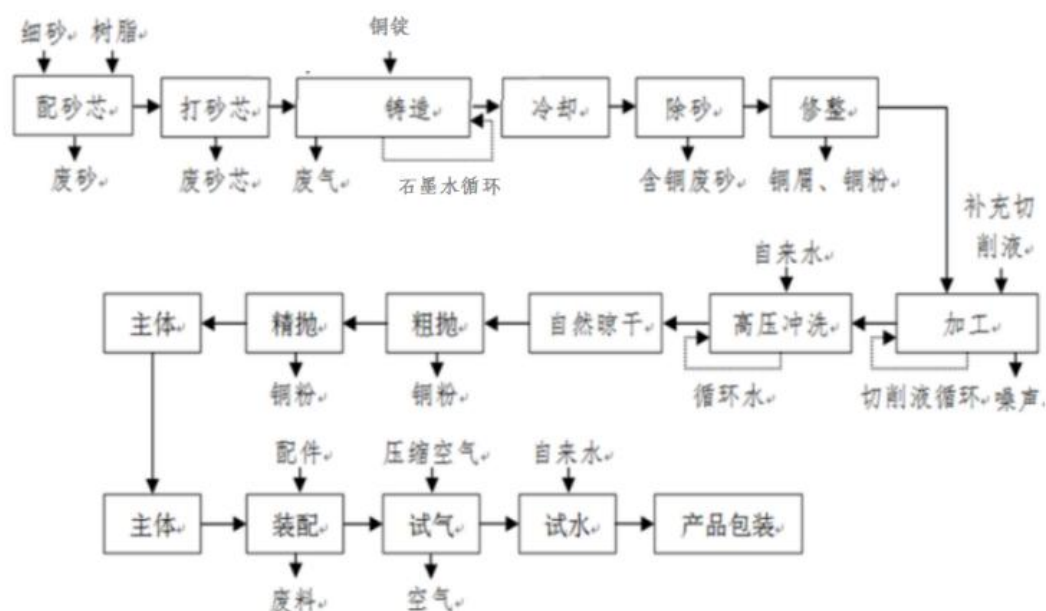
图 1-1 扩建前生产工艺流程图
