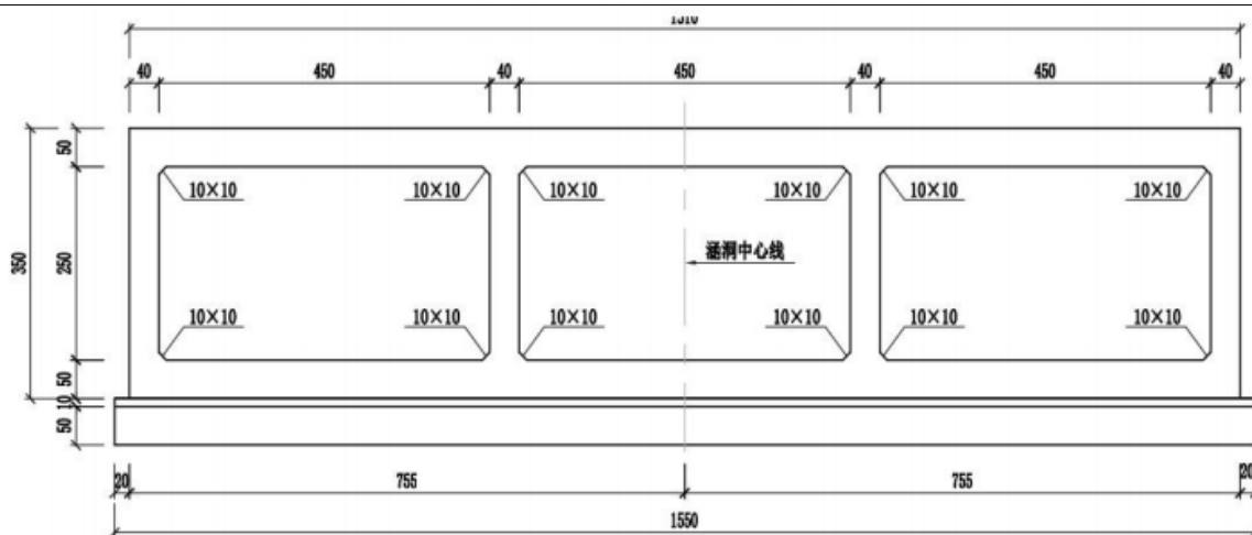
三孔箱涵横断面示意图 1:75
