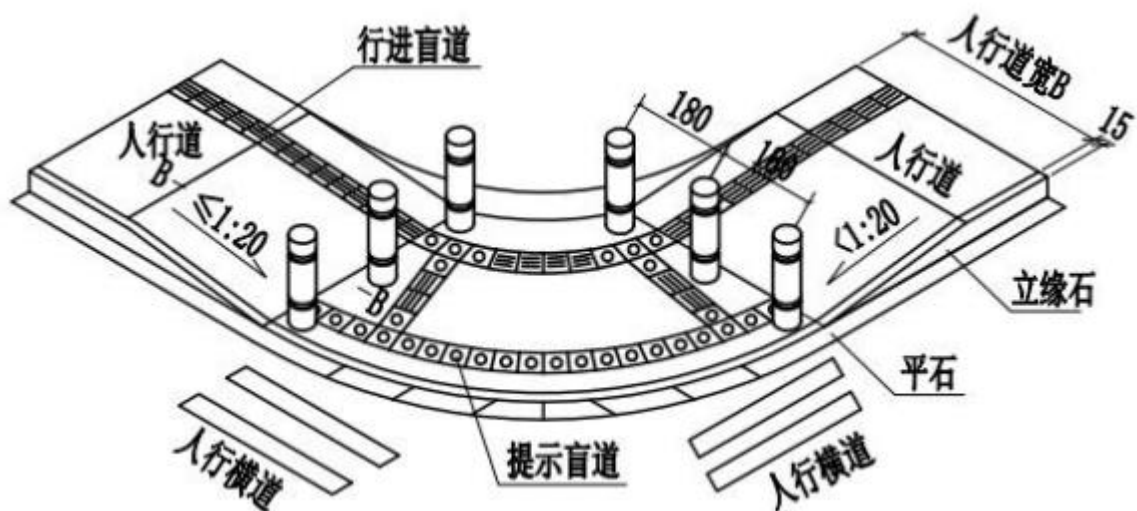
图 1-3 路口人行坡道平面位置图
