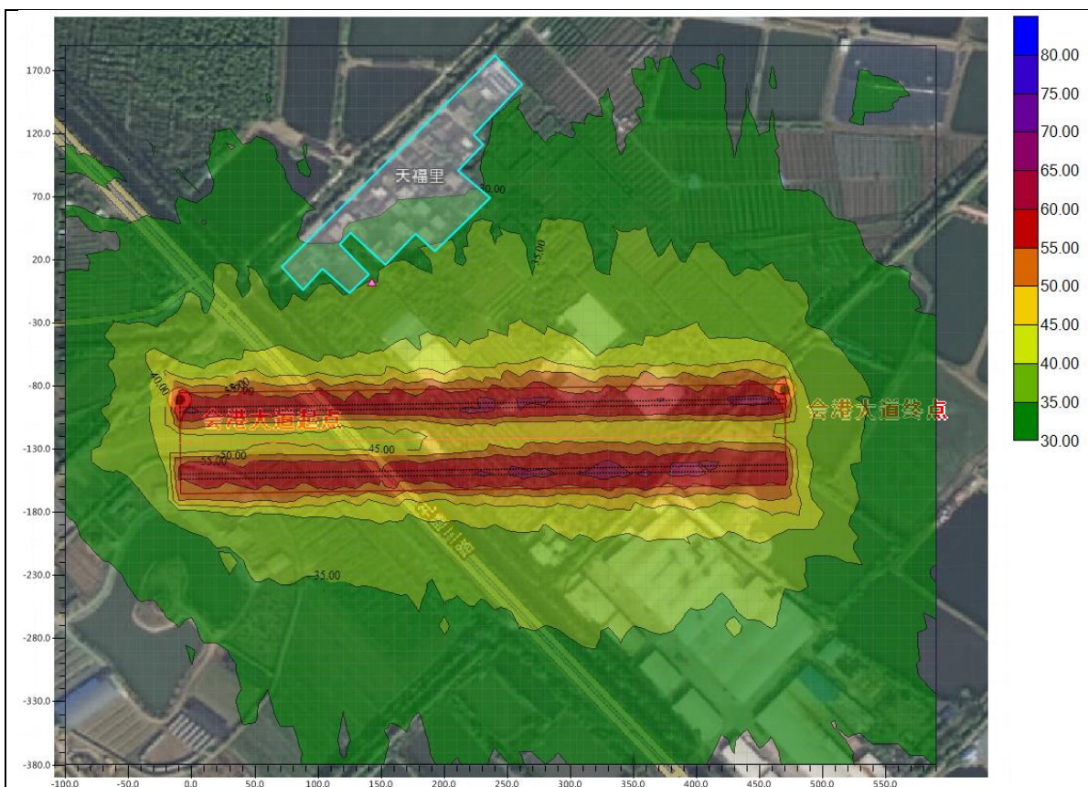
图 7-9 中期（2026 年）昼间等声级线图（单位：dB(A)）
