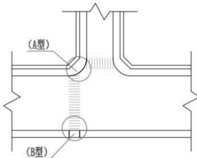
图 1-3 路口人行坡道平面位置图
