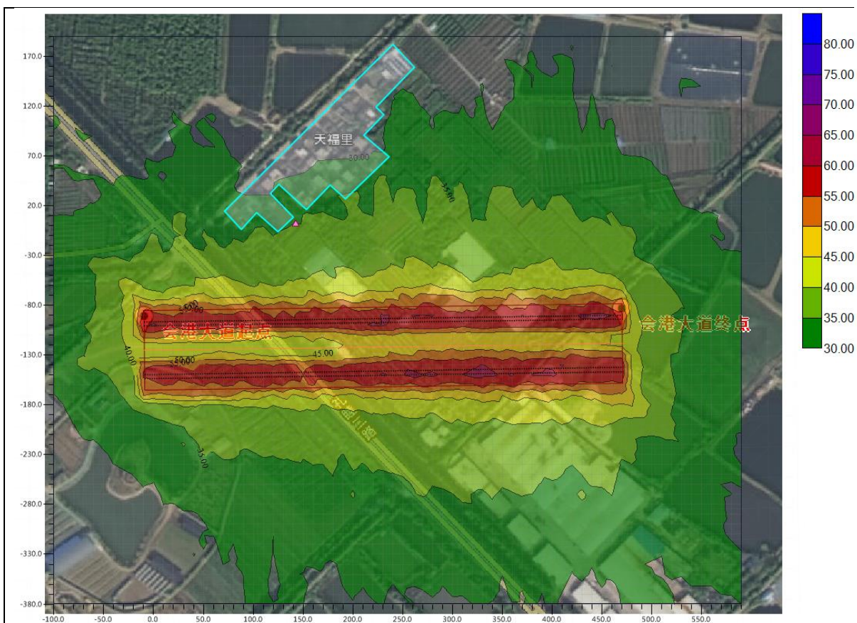
图 7-7 近期（2021 年）昼间等声级线图（单位：dB(A)）
