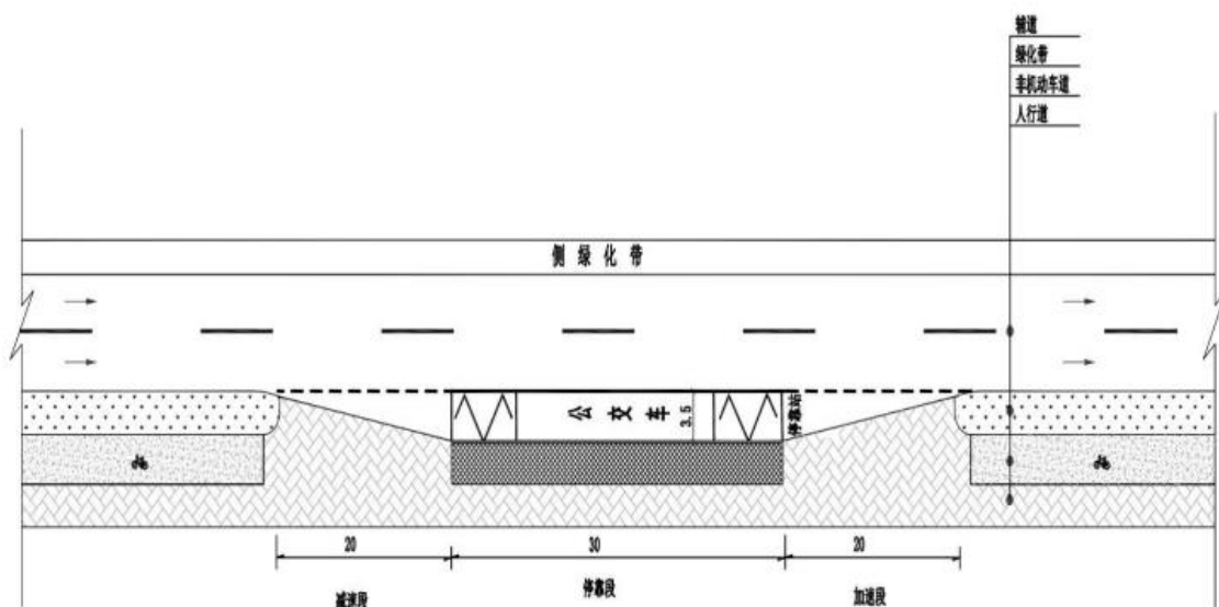
图 1-5 港湾式公交车停靠站
