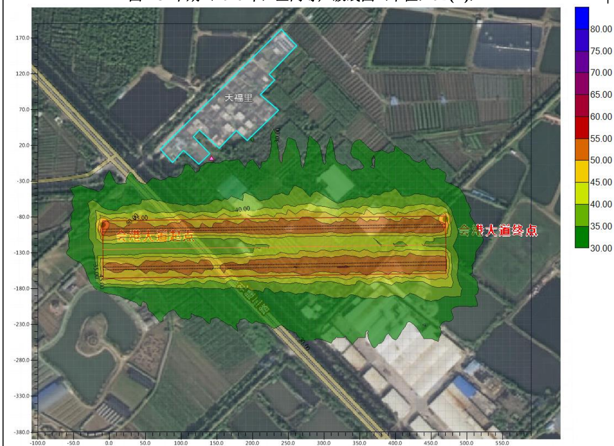
图 7-10 中期（2026 年）夜间等声级线图（单位：dB(A)）
