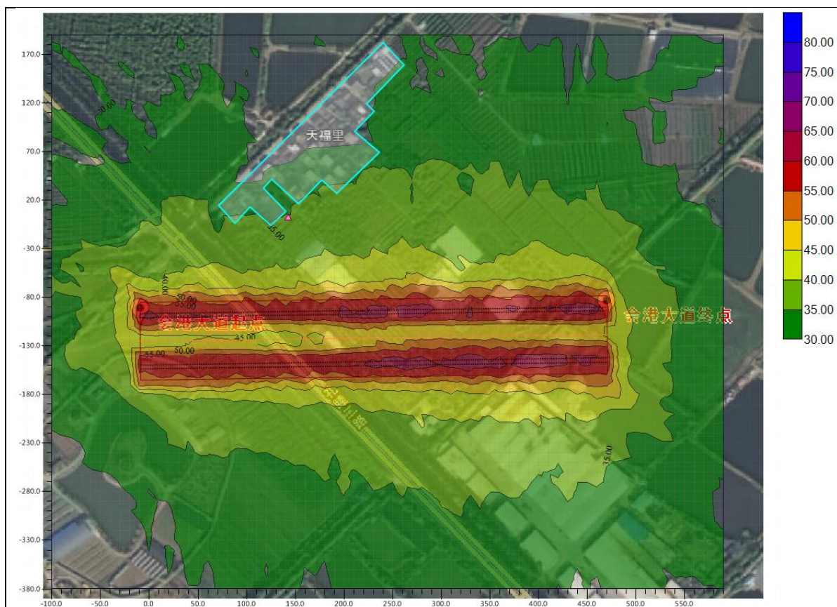
图 7-11 远期（2031 年）昼间等声级线图（单位：dB(A)）
