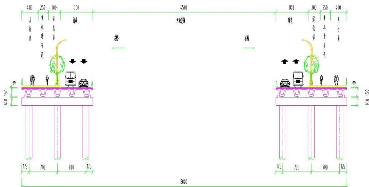
图 1-6 桥梁横断面图
