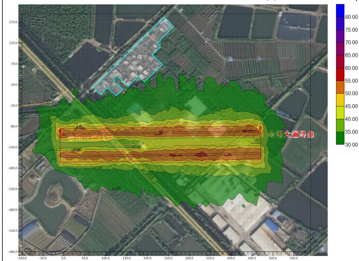
图 7-12 远期（2031 年）夜间等声级线图（单位：dB(A)）
