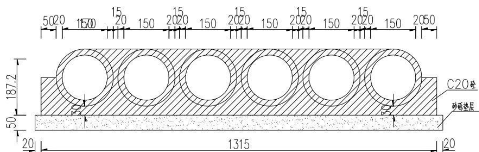
涵洞截面图
