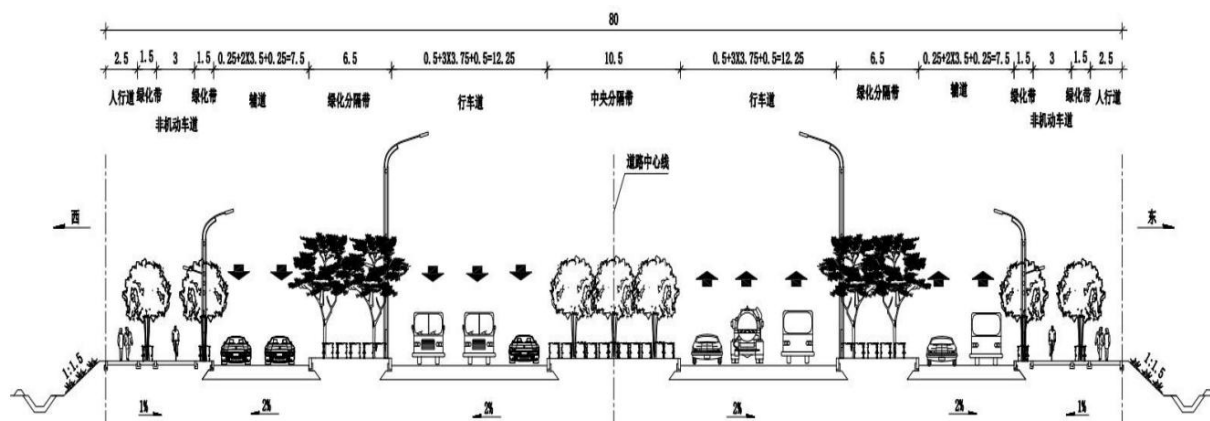
图 2-2 南山路道路横断面
