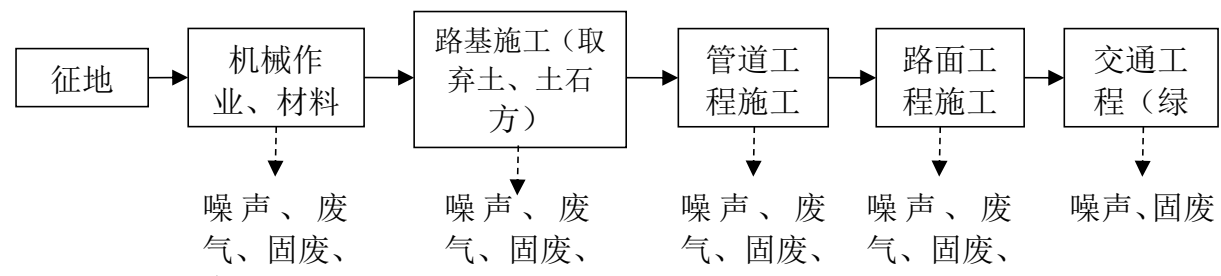
图 6-1 项目施工期工艺流程及产污环节图
