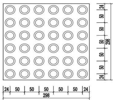
提示盲道砖块平面图
