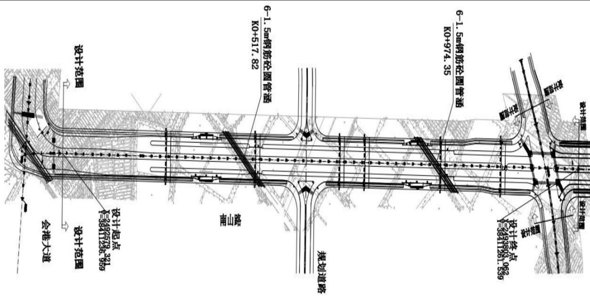
图 2-1 本项目总平面布置图
