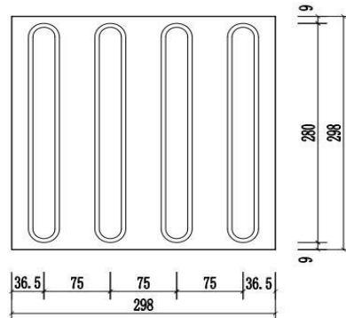
行进盲道砖块平面图
