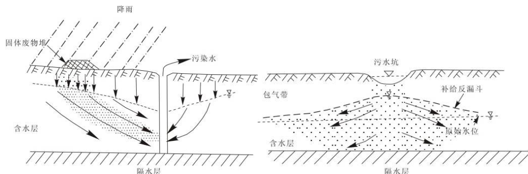
图 4-1 地下水间歇入渗型和连续入渗型简图
