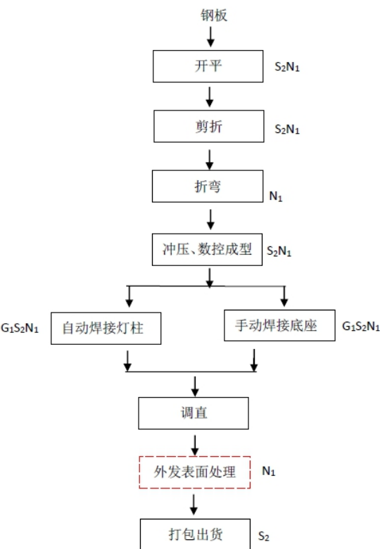
图 2-2 现有项目生产工艺流程图
