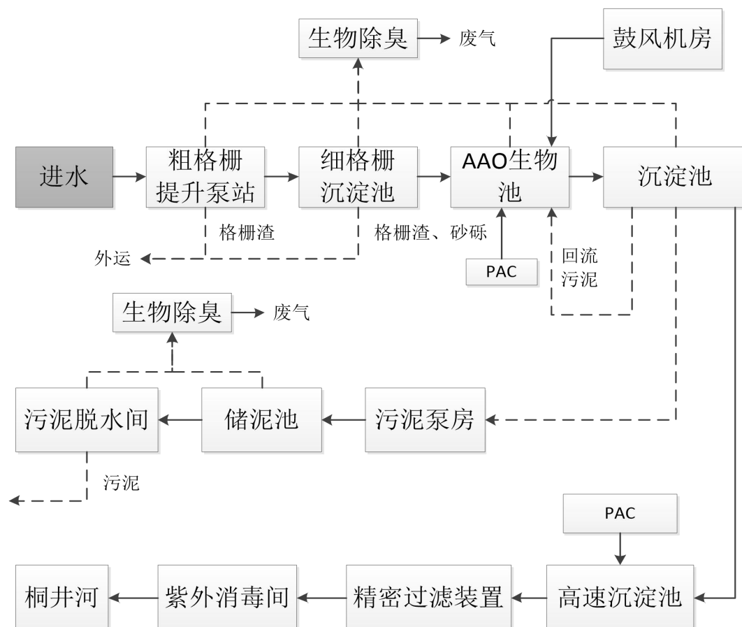
图 7.2-2 棠下污水处理厂处理工艺图
