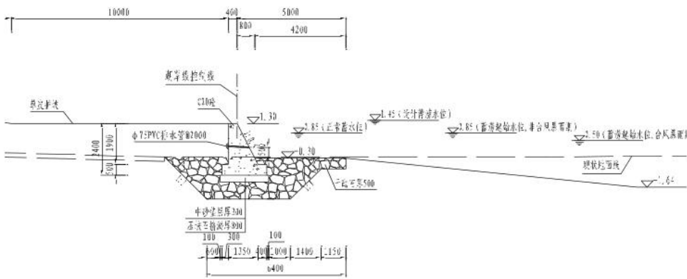
图 3.10-1 天沙湖、园山湖护岸挡土墙横断面图
