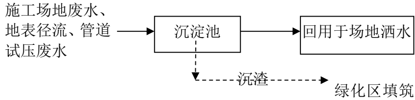
图 7.1-1 场地施工废水的处理工艺流程
