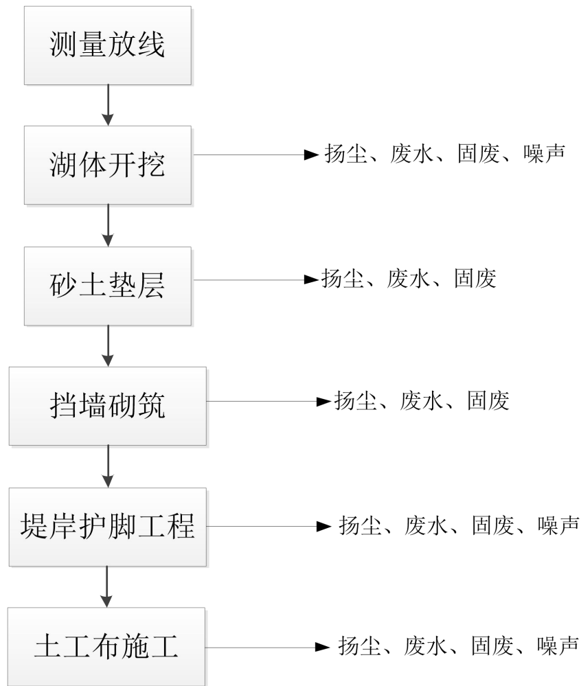
图 4.1-4 调蓄湖工程施工工艺流程
