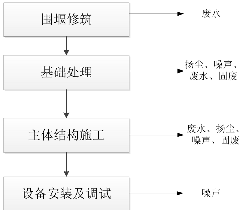
图 4.1-2 泵站施工工艺流程
