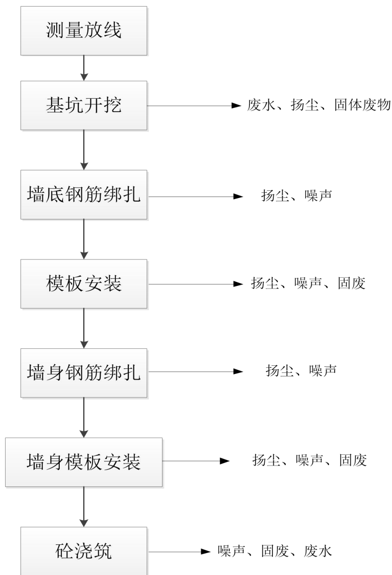
图 4.1-1 护岸挡土墙施工工艺流程
