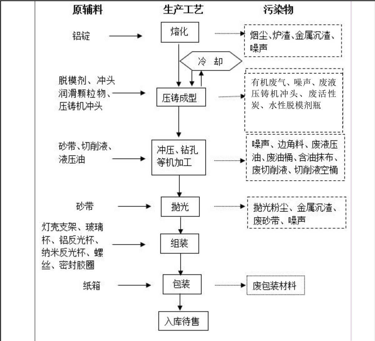
图 2-1 本项目生产工艺流程图
