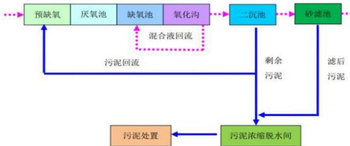
图 4-3 荷塘镇污水处理厂处理工艺流程图
