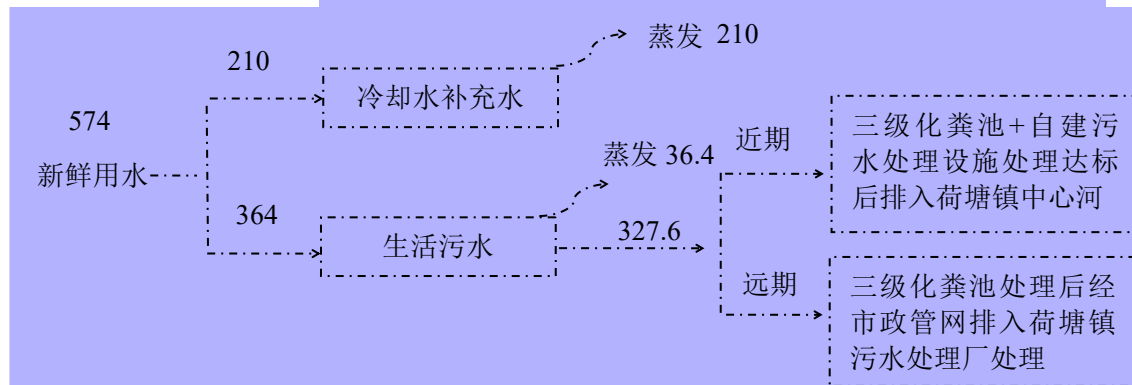
图2-1 项目水平衡图 ( \text{m}^3/\text{a} )
