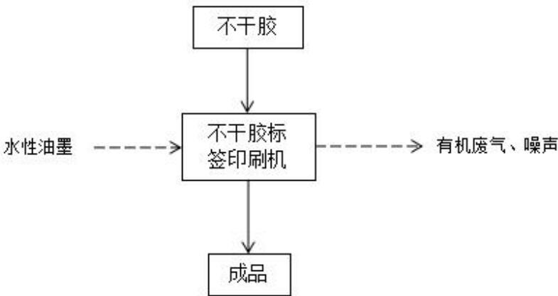
图 2-1 不干胶标签纸印刷工艺流程图
