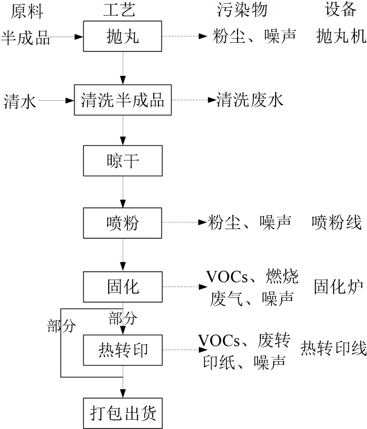
图2-2 项目营运期生产工艺流程及产污环节
