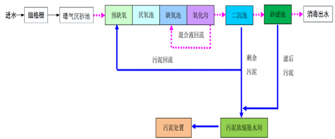
图 4-1 荷塘镇生活污水处理厂工程工艺流程
