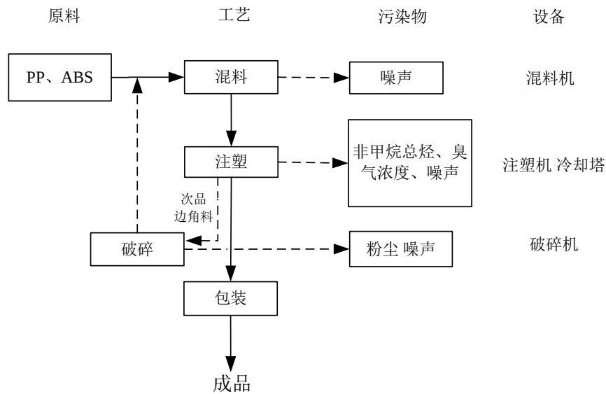
图2 生产工艺流程图
