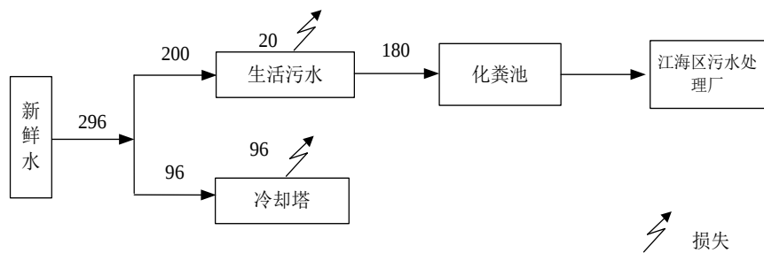
图1 项目水平衡图（t/a）
