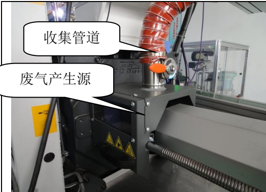
注塑废气收集图 1
