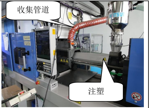
注塑废气收集图 2
