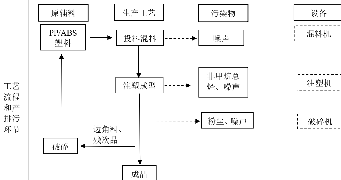
图 2-1 项目生产工艺流程图
