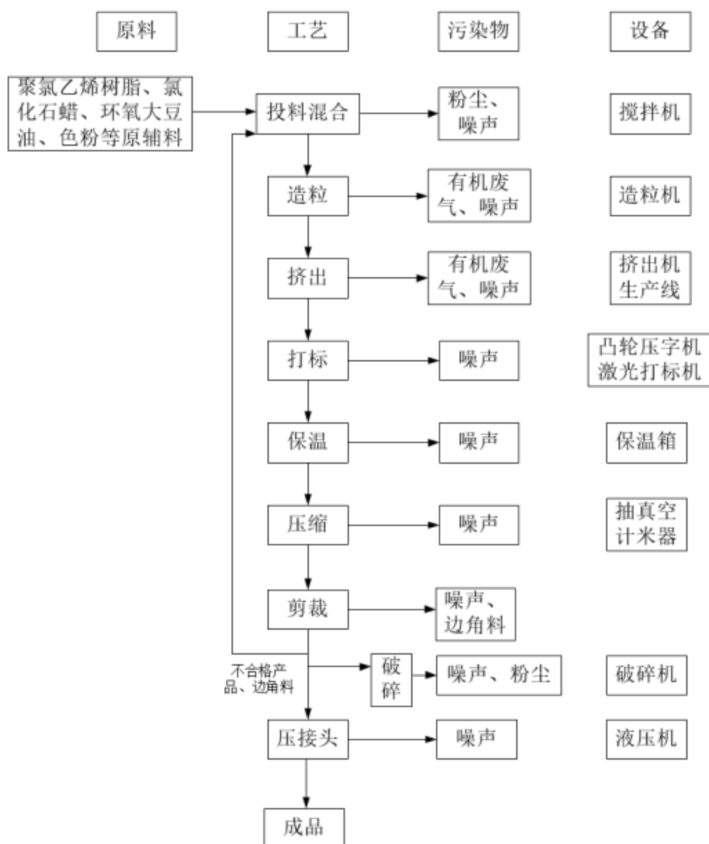
图 2-2 生产工艺流程及产污环节示意图
