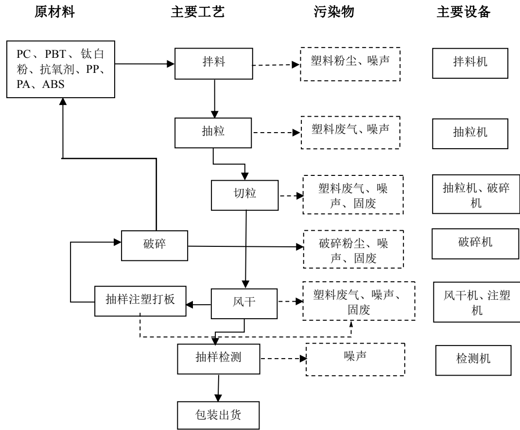
图 2-2 产品生产工艺流程图
